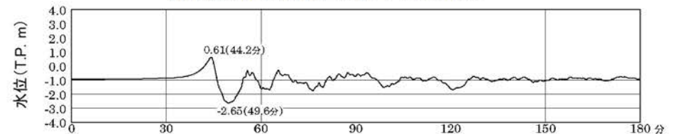
【水位下降側：3, 4号炉取水口位置】 対馬南西沖断層群と第1五島堆断層帯の連動 (初期潮位：L.W.L.(T.P.-0.98m))
