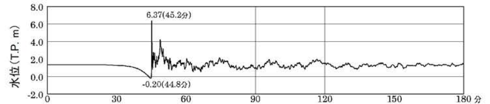
【水位上昇側：3, 4号炉取水ピット前面位置】 対馬南西沖断層群と第1五島堆断層帯の連動 (初期潮位：H.W.L.(T.P.+1.31m))
