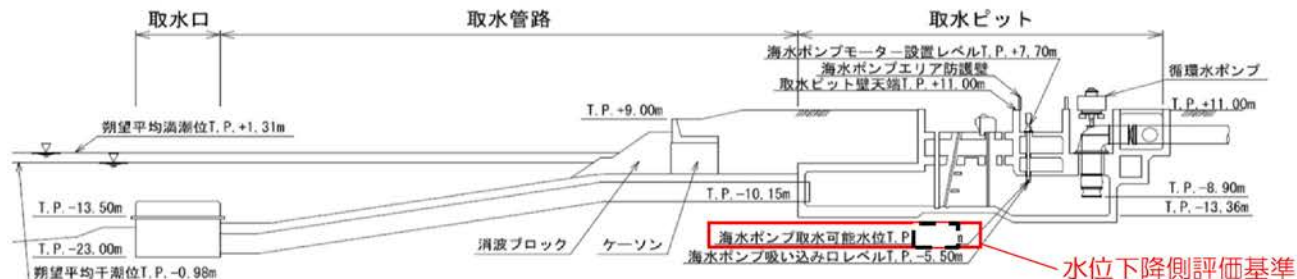
水位下降側評価結果(対馬南西沖断層群と第1五島堆断層帯の連動、循環水ポンプ運転時)
