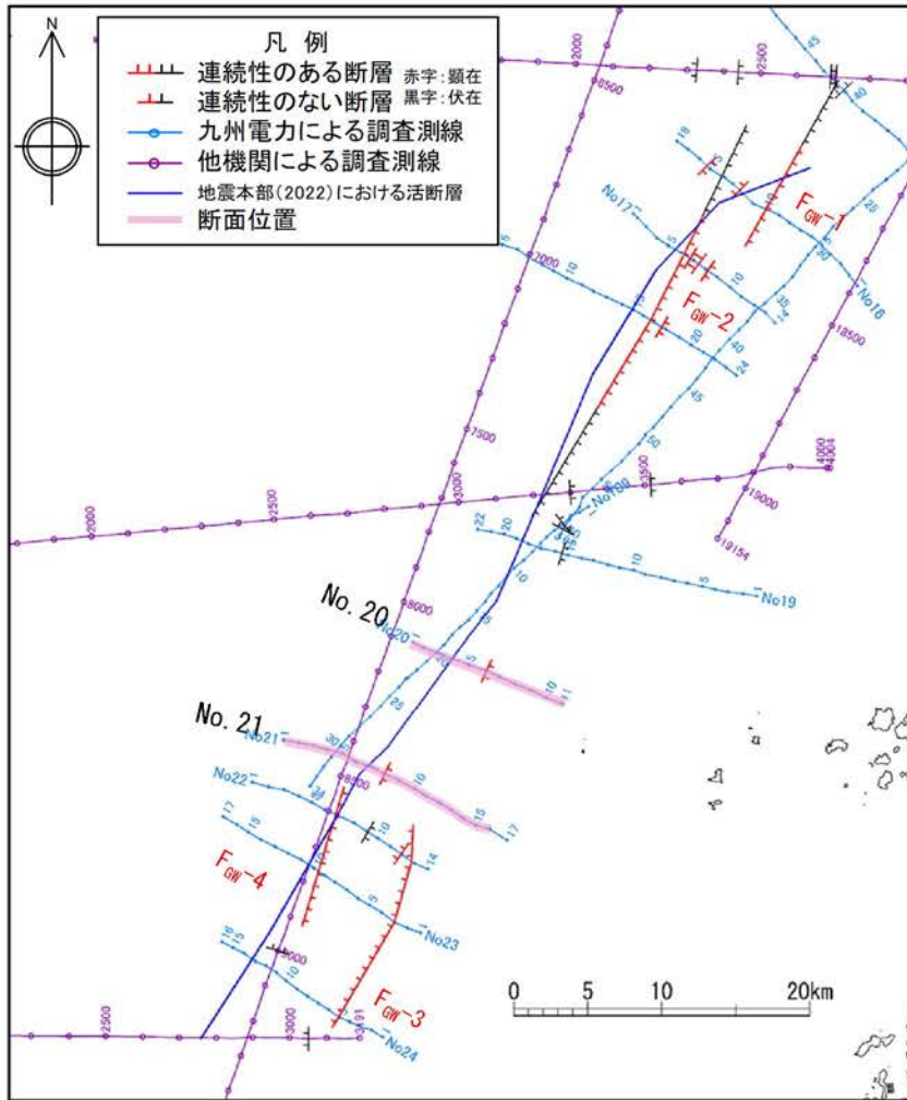
断層分布図
