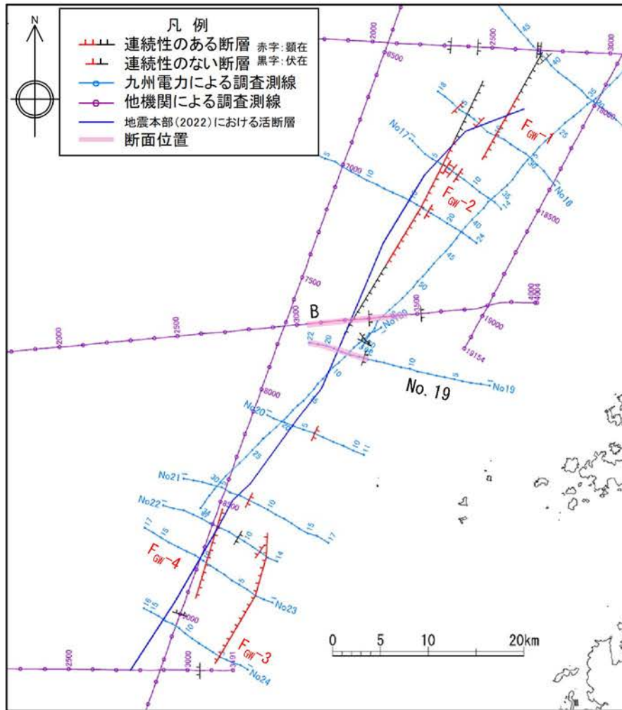
断層分布図
