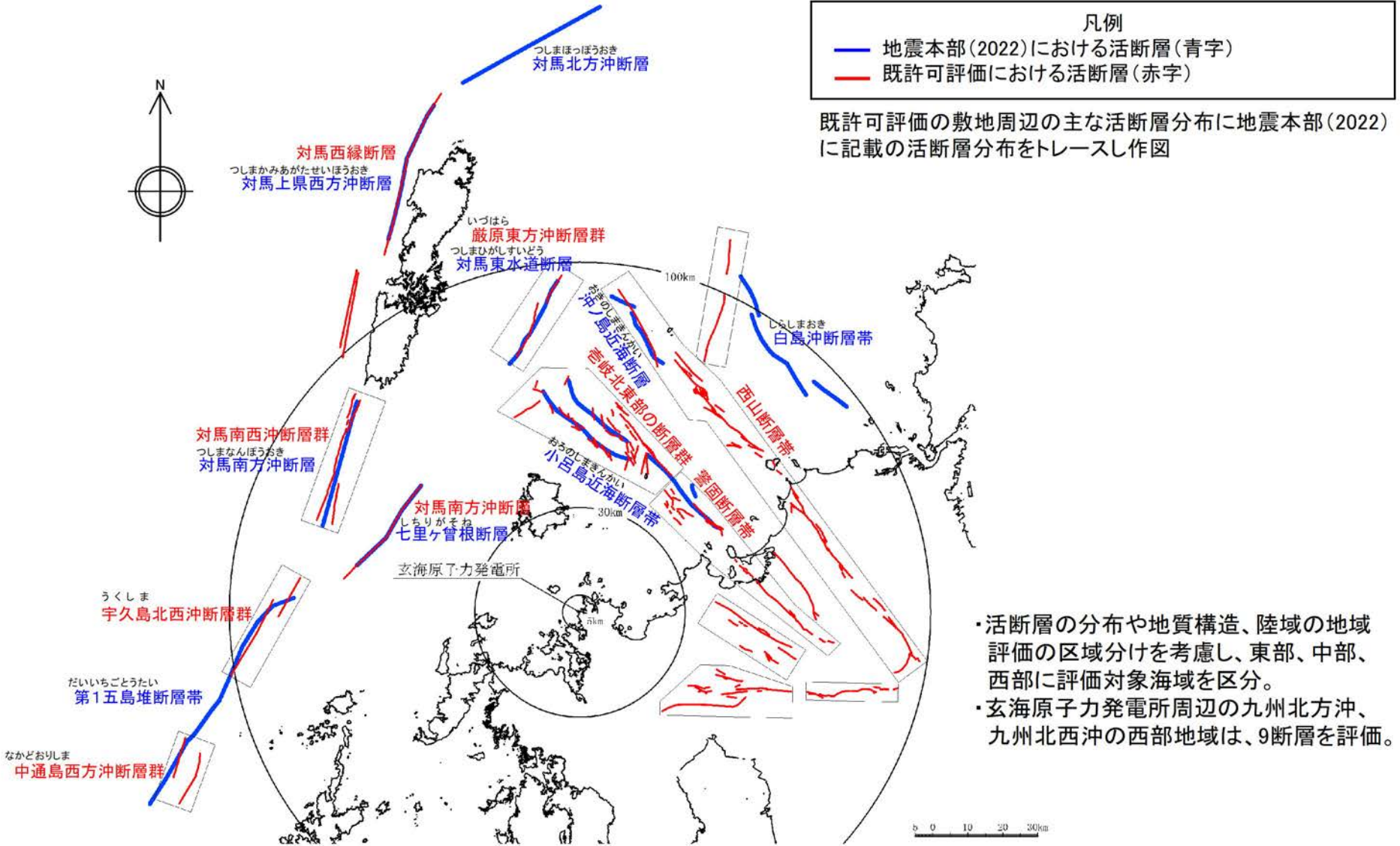
敷地周辺の主な活断層分布(敷地30km以遠)
