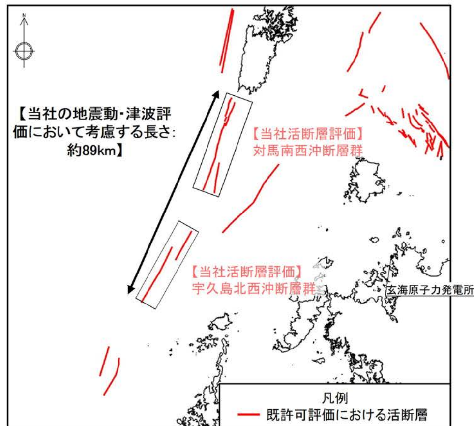
既許可評価における断層分布図
