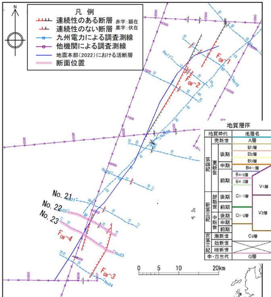
断層分布図
