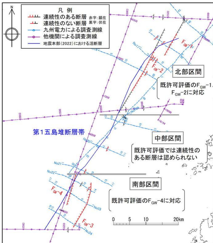
断層分布図
