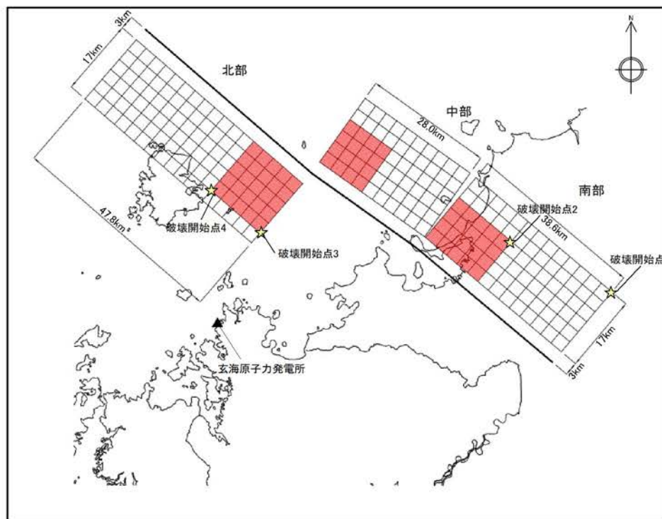
震源モデル
