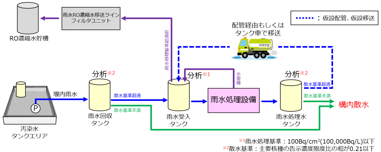
図 2.9-2 概略系統図(通常の処理方法)
