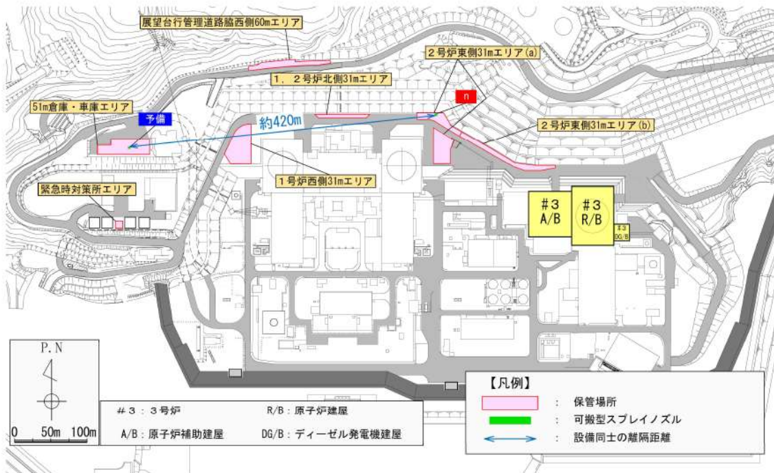
可搬型スプレイノズルの相互の離隔距離
