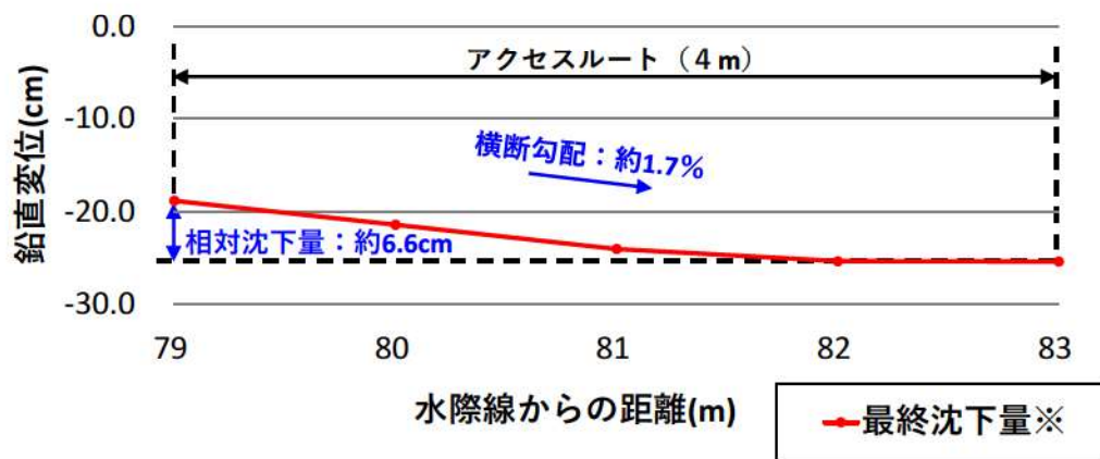
図7-27 側方流動を考慮した地表面変位評価結果 (アクセスルート)
