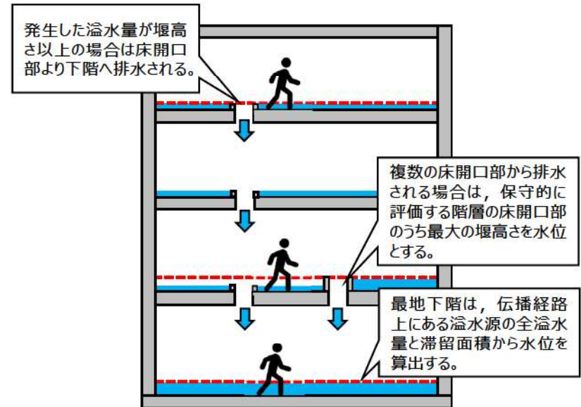
図9-5 洪水水位評価概要図
