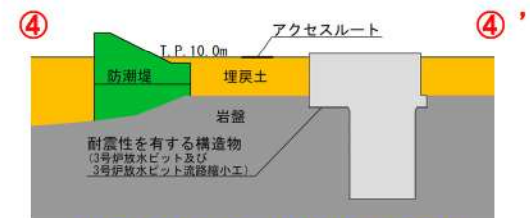
図7-25 ④-④'地点断面図
