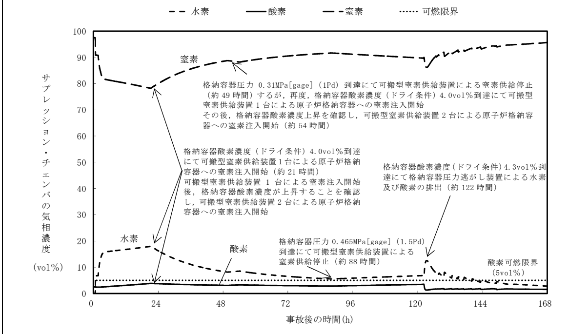
第 2 図 「雰囲気圧力・温度による静的負荷 (格納容器過圧・過温破損) (代替循環冷却を使用する場合)」において可燃性ガス濃度制御系の性能評価で使用している G 値を採用した場合のサブプレッション・チェンバの気相濃度の推移 (ドライ条件)
