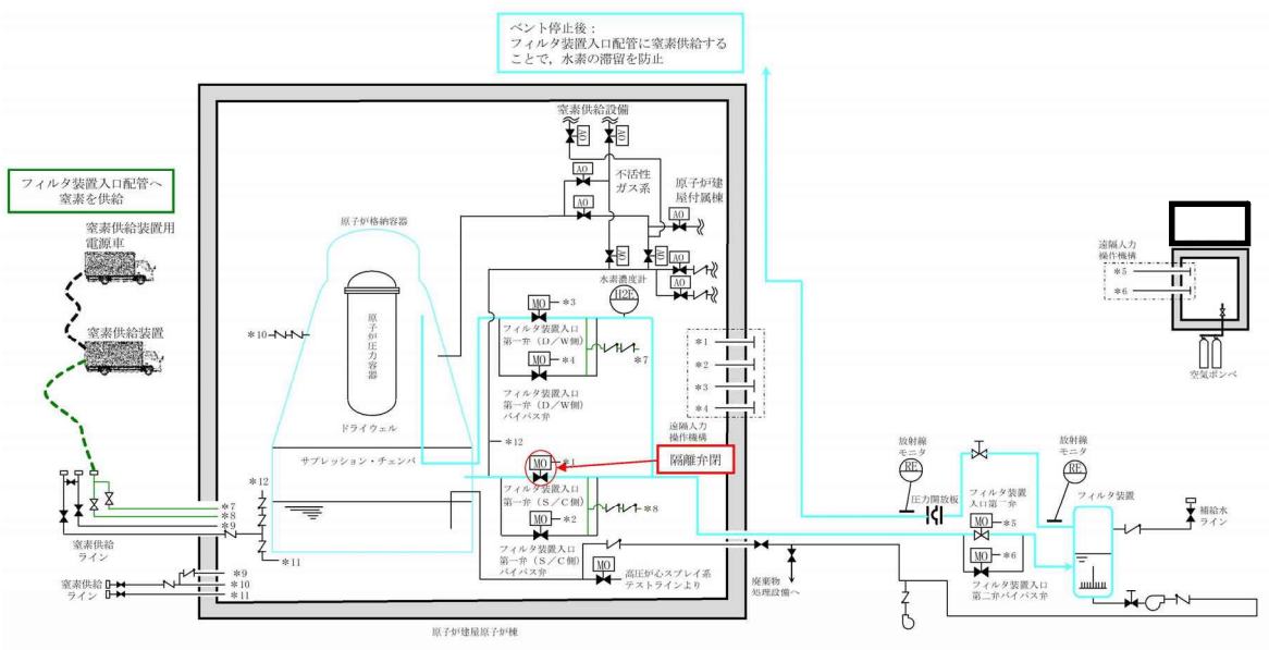
第 4.1.3-8 図 室素供給概要図 (ベント停止後)
