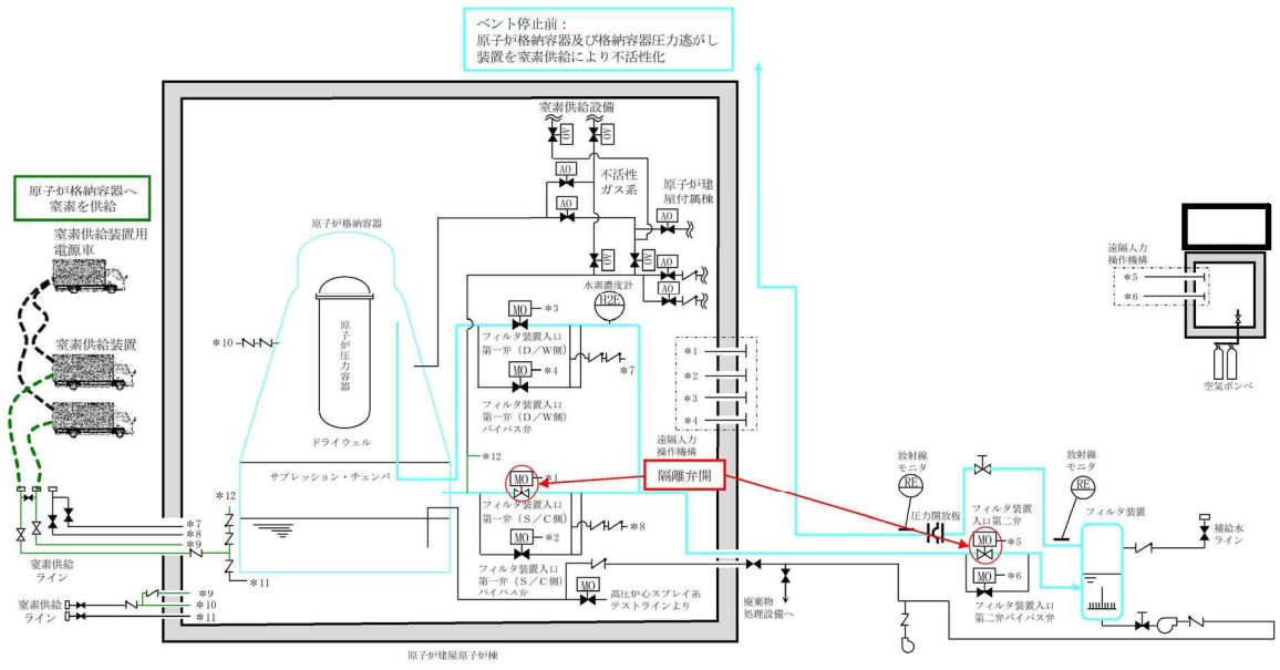
第 4.1.3-7 図 室素供給概要図 (ベント停止前)
