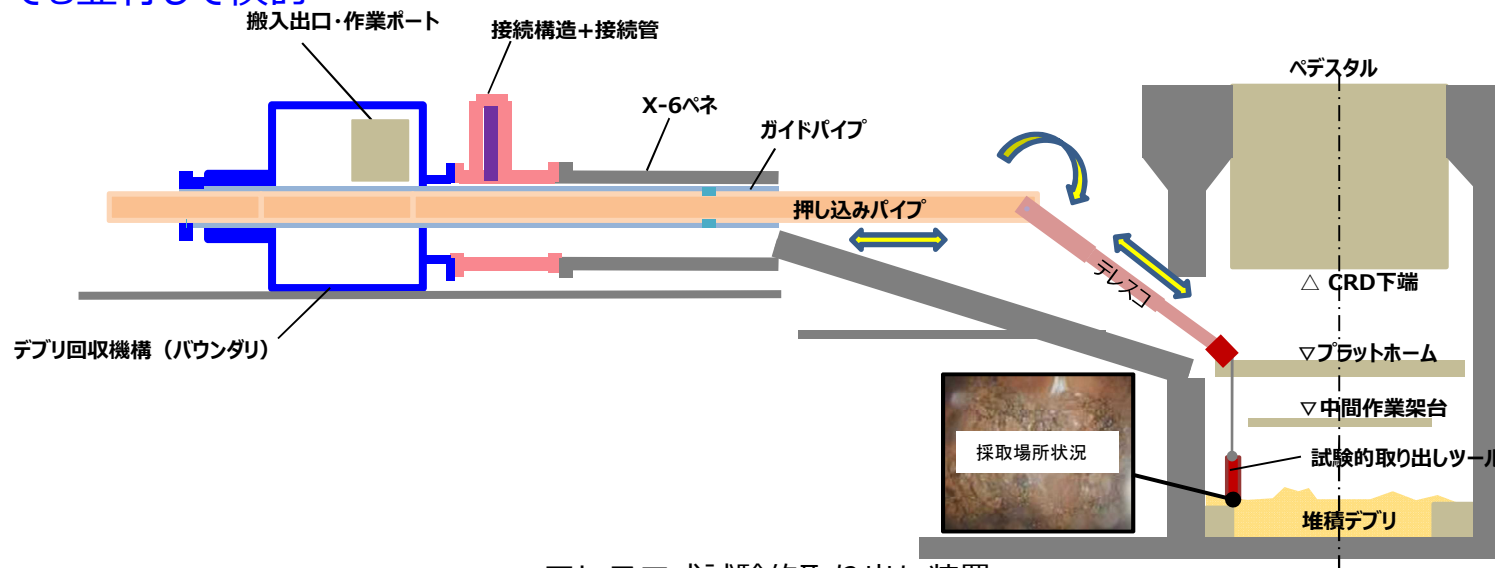
テレスコ式試験的取り出し装置
