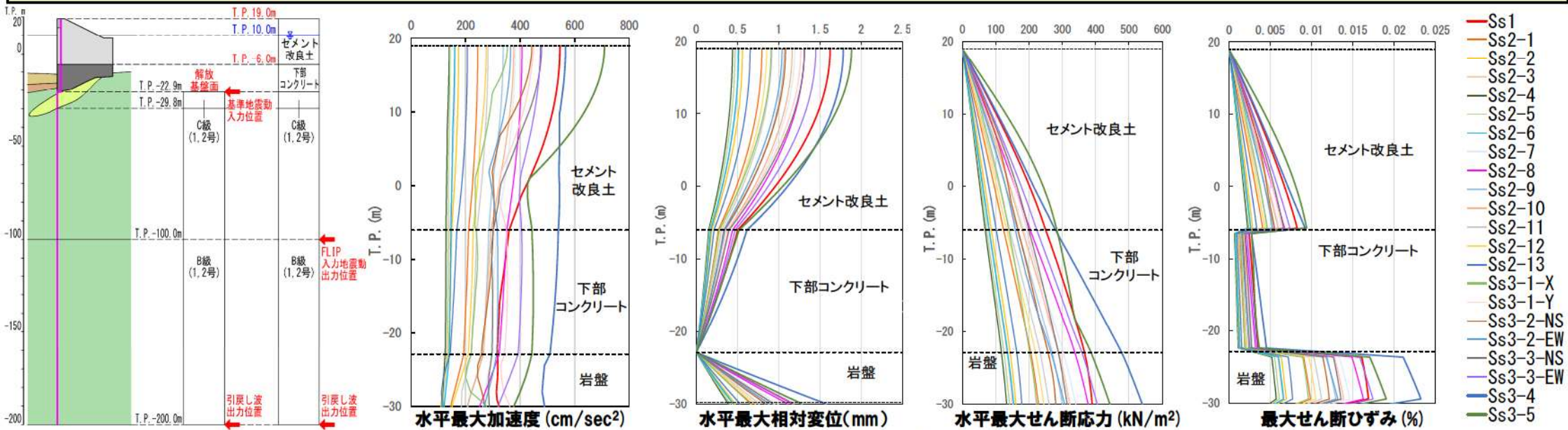
1次元波動論による地震応答解析モデル (「2-2'断面」の防潮堤前面位置※1)
