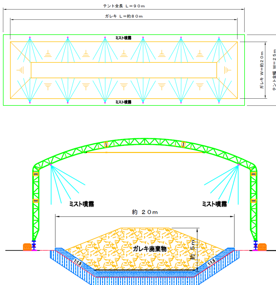
図 2.11-1 覆土式一時保管施設を覆うテントの概略図
