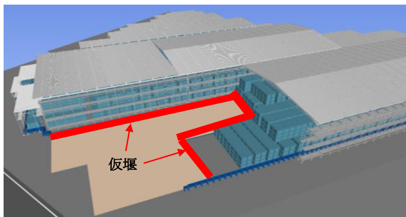
図 2.9-1 作業期間における仮堰の設置状況
