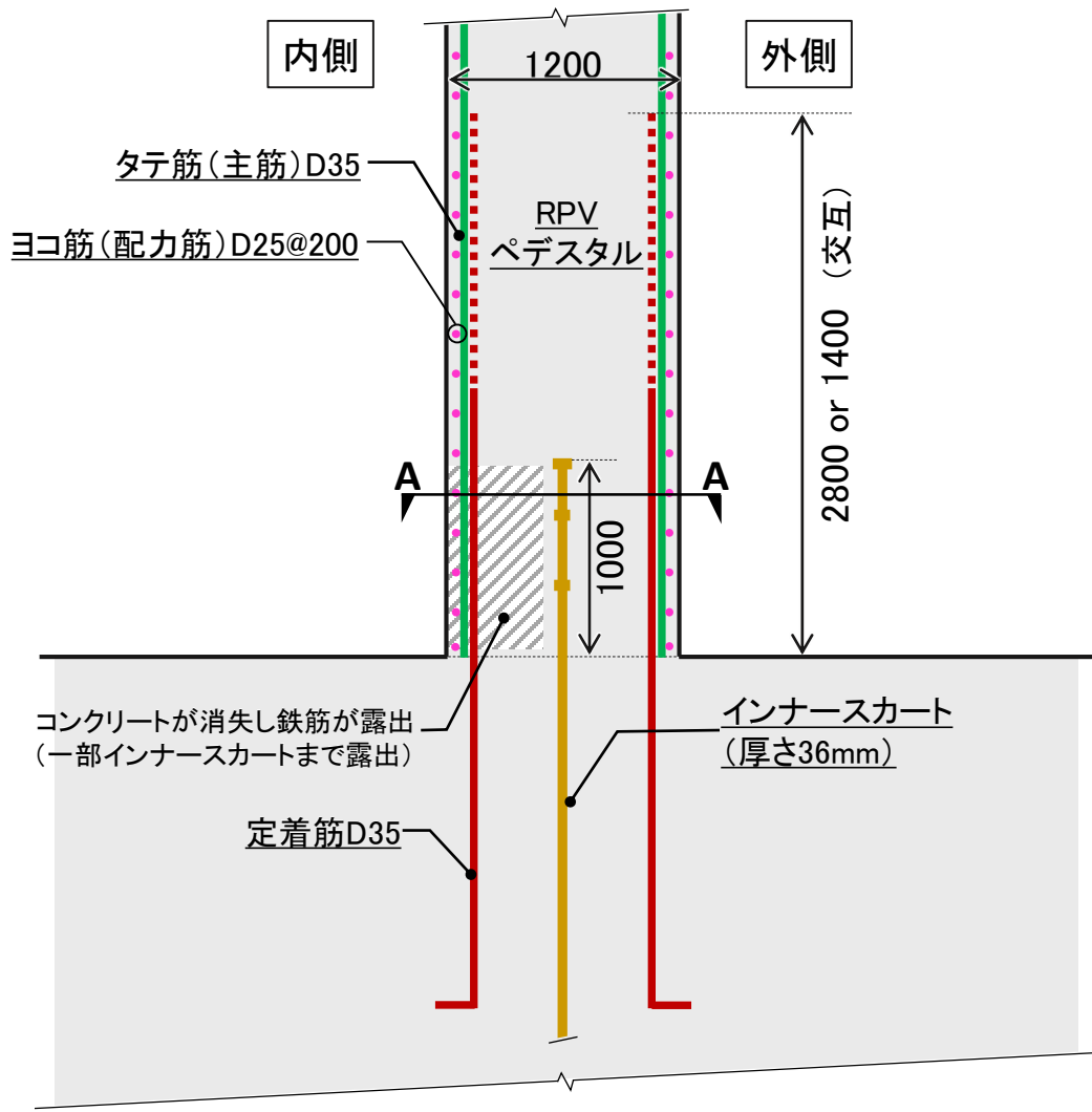
ペDESTAL基部 断面イメージ
