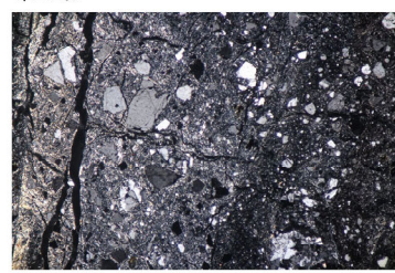
直交ニコル
