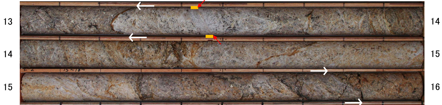
コア写真
