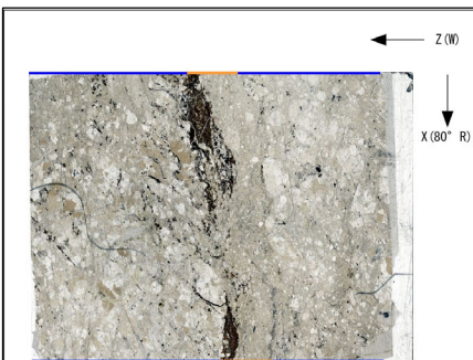
単ニコル
