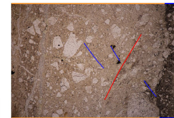
単ニコル
