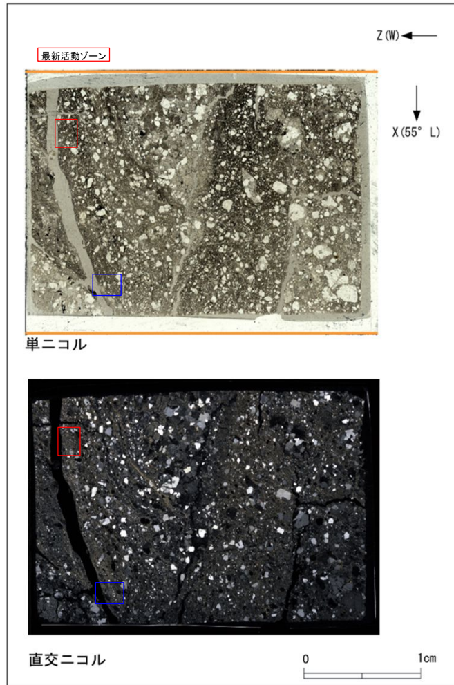
単ニコル
