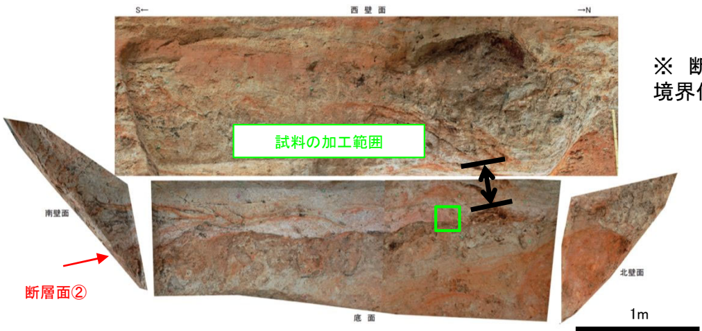
露頭写真
