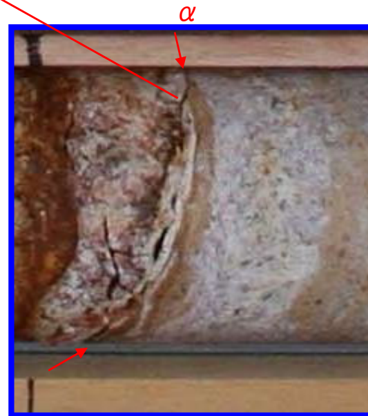
青枠部拡大
