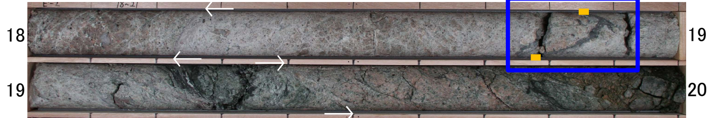
コア写真
