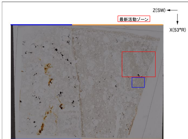
単ニコル
