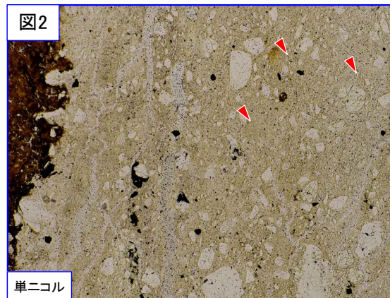
赤三角印の方向は粘土鉱物の配列方向を示す
