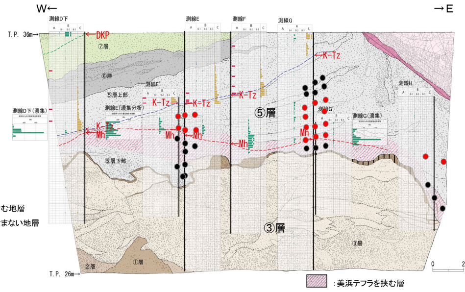
粒度分析用試料採取位置図(D-1トレンチ北法面)
