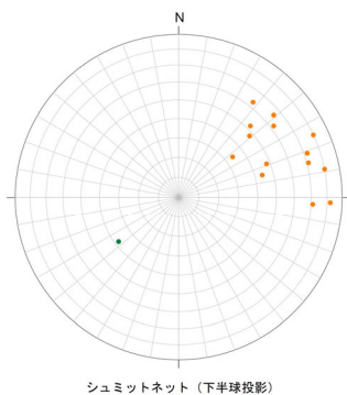
シュミットネット (下半球投影) ● せん断面 (K断層) : 16 ● 断層面 : 1
