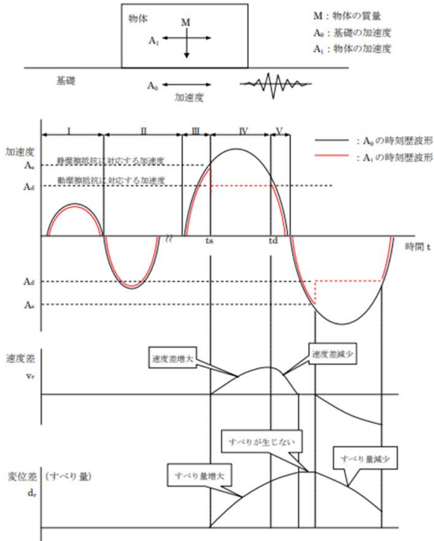
図 2.14.2.2-3 Newmark 法の概要
