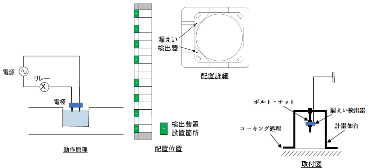
図 2.14.1-8 漏えい検出器の動作原理，設置状況
