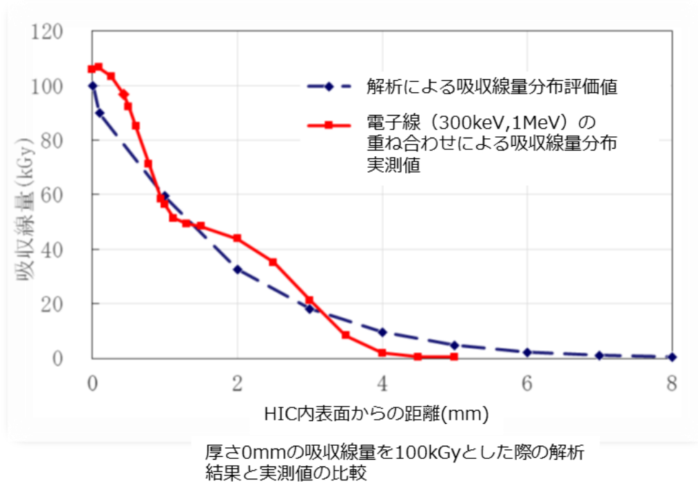
図 2.9.1-3 電子線による吸収線量分布実測値
