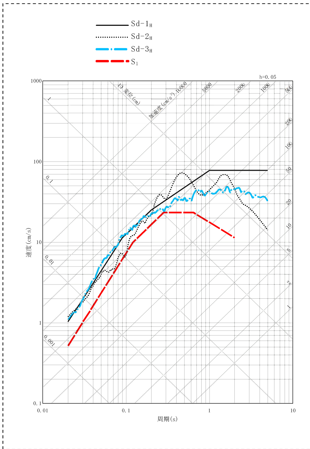
第 1.4.6 図 弾性設計用地震動と基準地震動 S 1 の応答スペクトルの比較 (水平方向) 注 3
