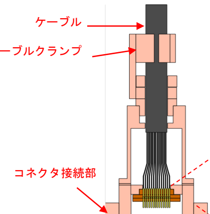
テレスコ側コネクタ部詳細 (正常)
