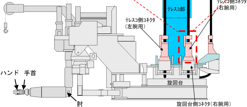
図-6 両腕型マニプレータ_G51M120側面図
