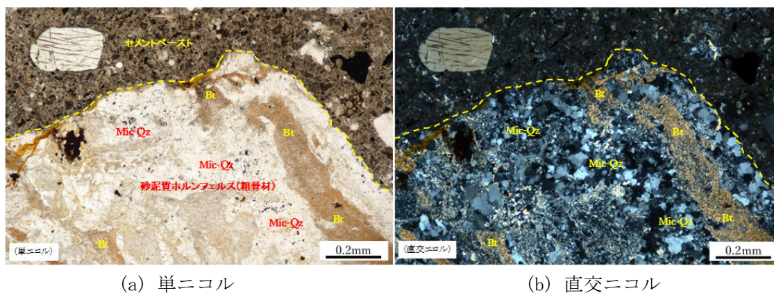
図 1 粗骨材の偏光顕微鏡観察写真
