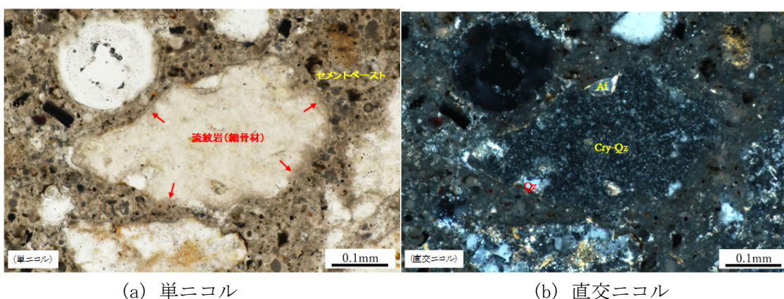
図 2 細骨材（チャート）の偏光顕微鏡観察写真
