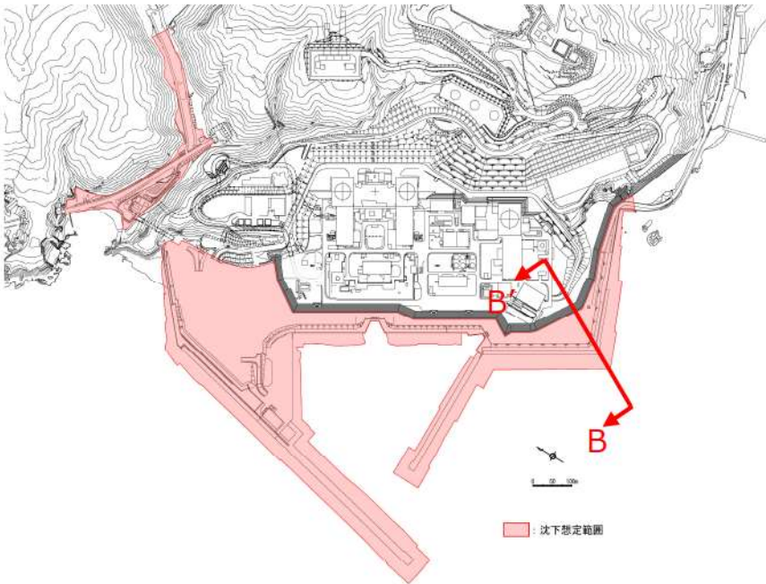
敷地地盤(陸域)の地盤変状として沈下を考慮する範囲
