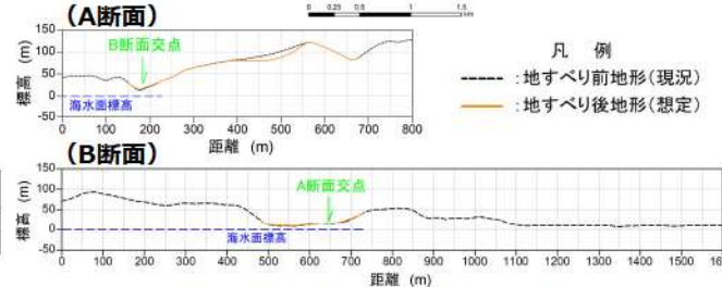
地滑り地形③による地形変化量
