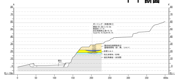
A-A' 断面
