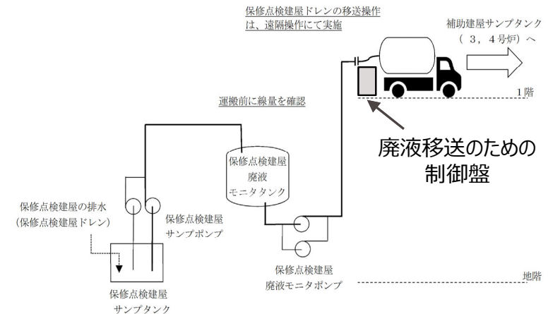
図2 廃液の運搬容器への移送
