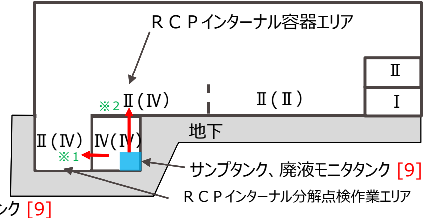
図2 立面図 (A-A'断面)
