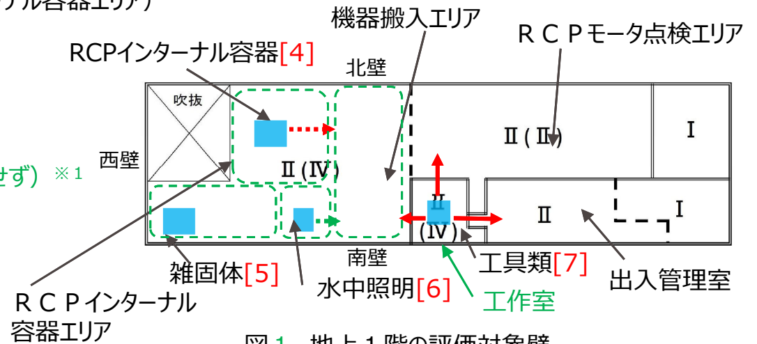
図1 地上1階の評価対象壁
