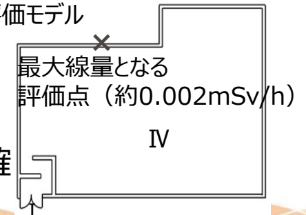
図 3 遮蔽設計区分概要図
