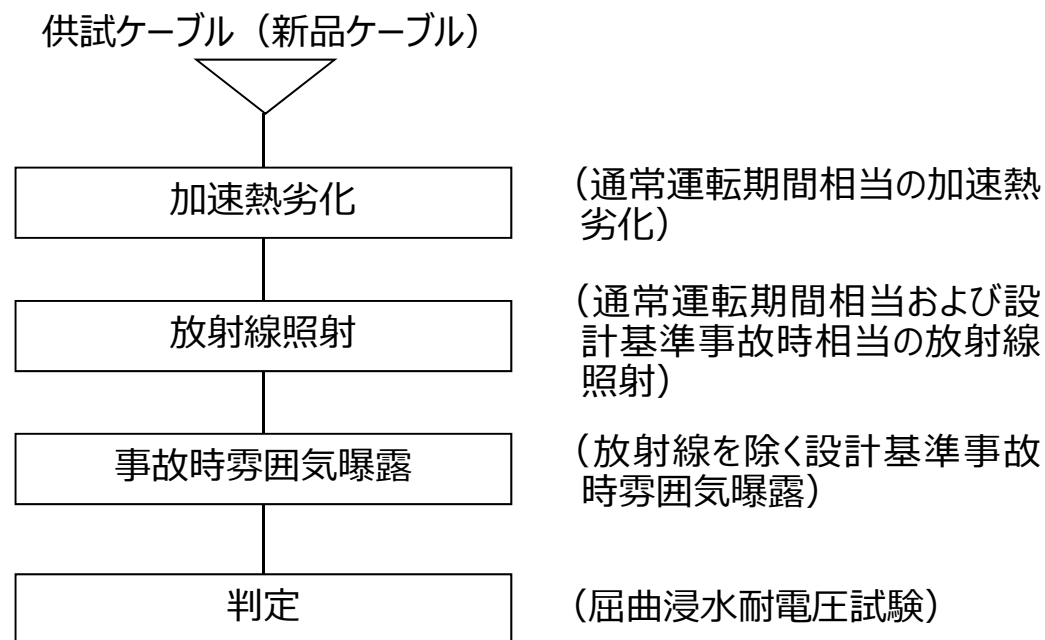
難燃PNケーブルの長期健全性試験手順
