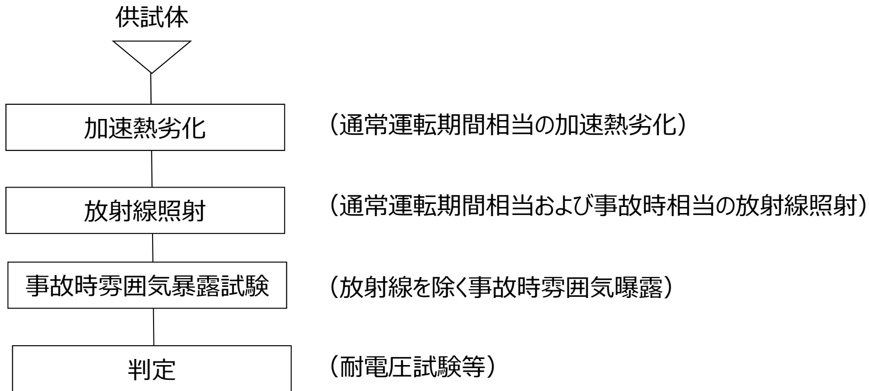
図 1 IEEE・電気学会推奨案による健全性評価手順
