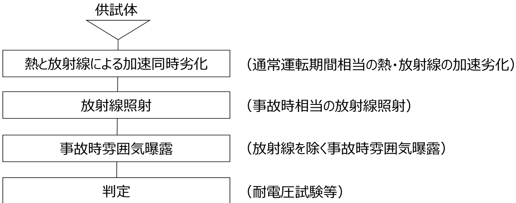
図2 ACAガイドによる健全性評価手順
