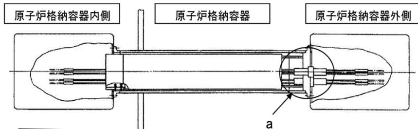
核計装用電気ペネトレーションの構造図
