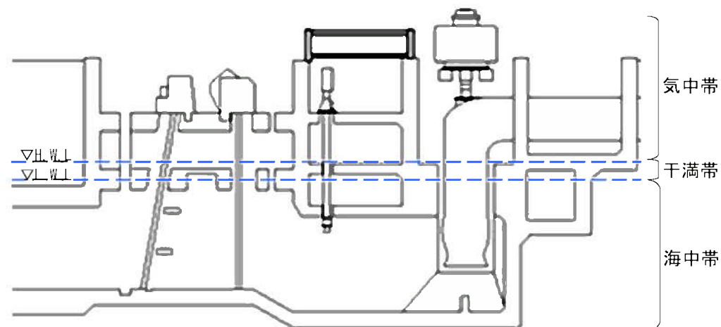
断面図 取水構造物[コンクリート構造物] ( H.W.L.: T.P. +1.31m L.W.L.: T.P. -0.98m )
