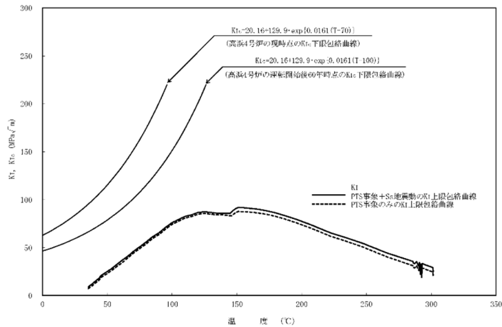
図 7-2 Ss 地震を考慮した PTS 評価結果 (想定亀裂深さ 10mm)
