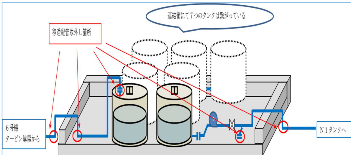
図4 6号機タービン建屋移送ポンプ接続図
