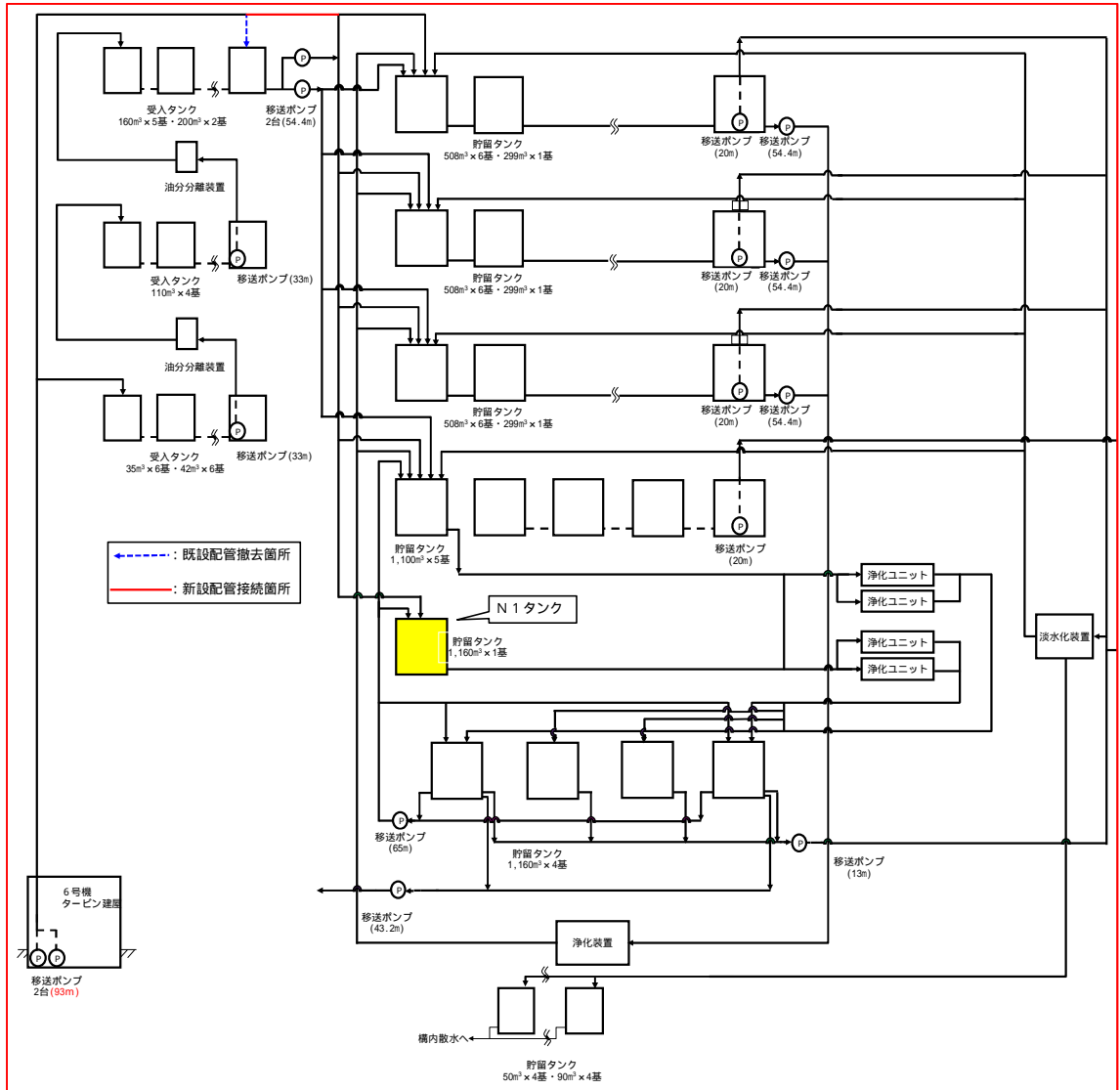
図3 系統概略図
