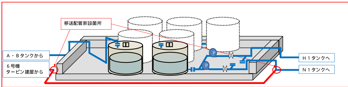
図6 5・6号機滞留水移送配管新設予定図
