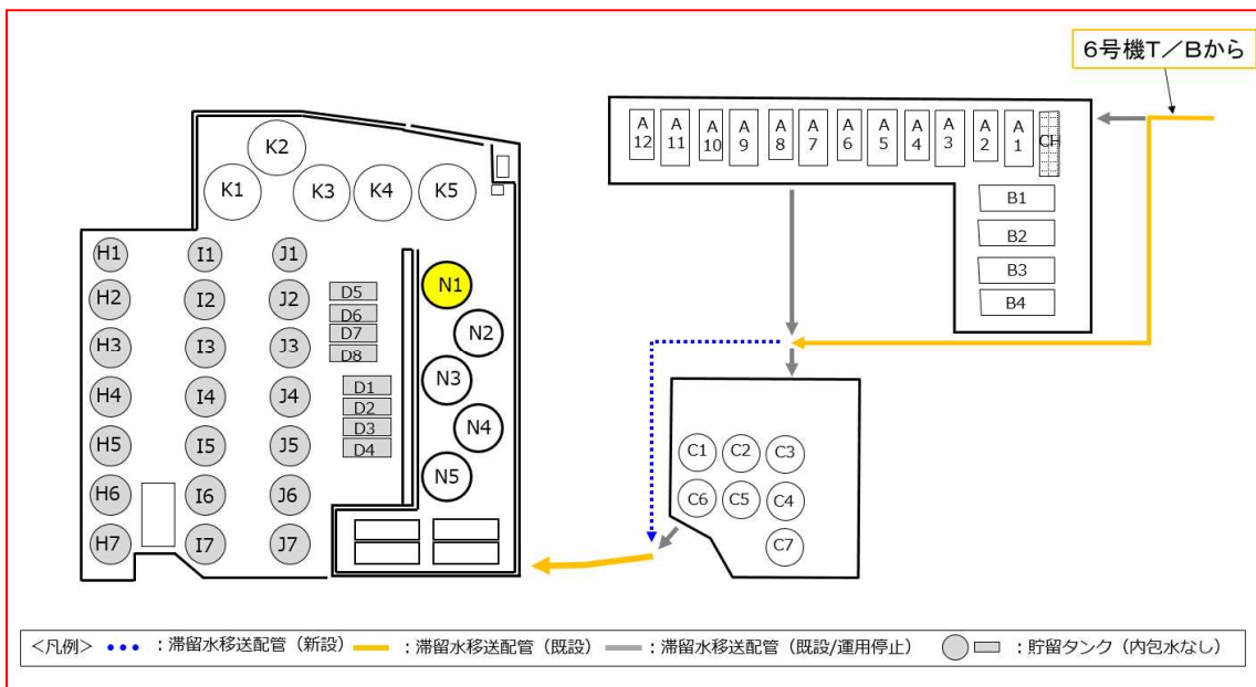
図 1 - 4 5・6号機滞流水移送設備の全体系統図 (詳細)
