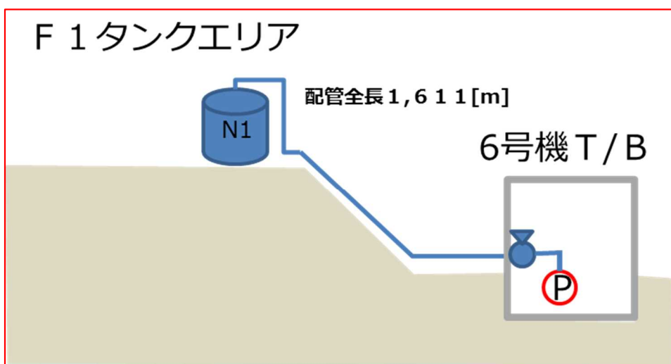
図1 5・6号機滞留水移送配管の水撃評価
