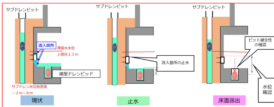
図2 5・6号機滞留水低減対策
