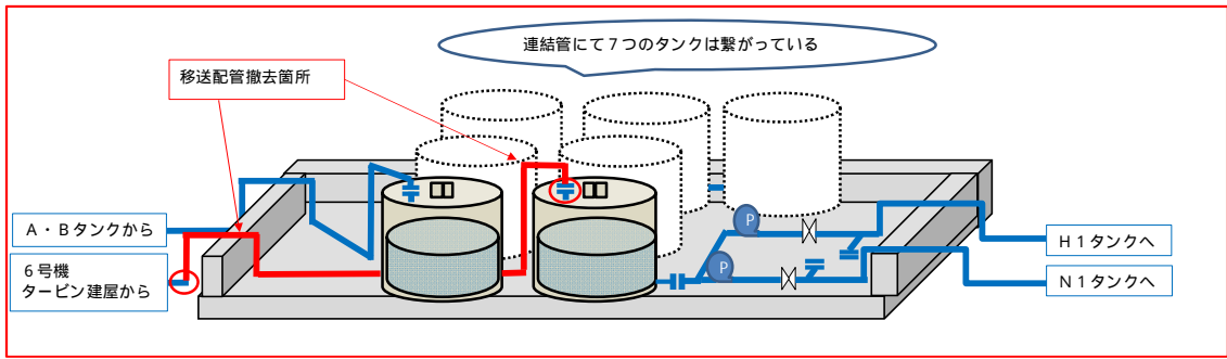
図4-5 5・6号機滞留水移送配管継ぎ手部取外し箇所
