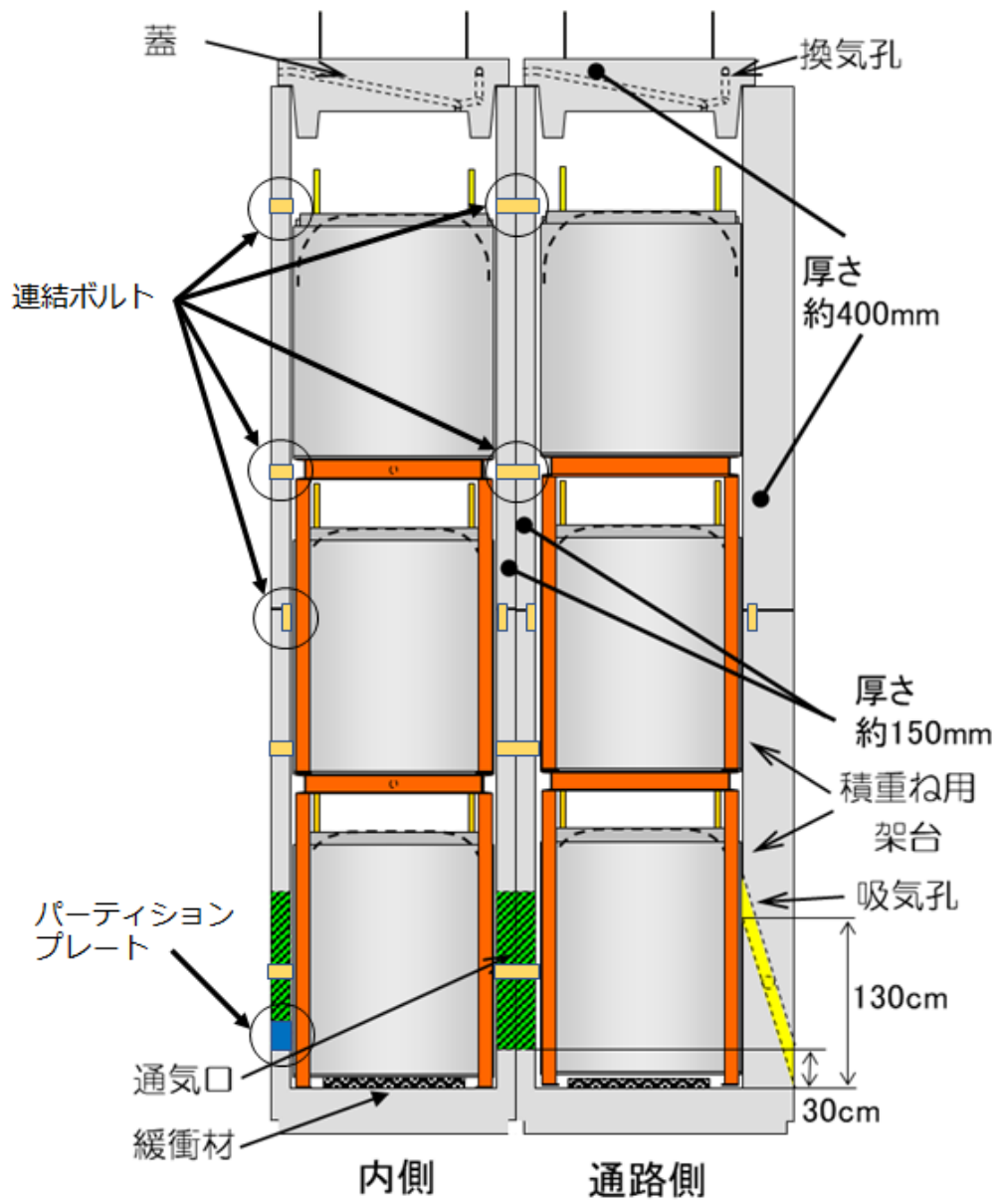
図 2.14.1-1 ボックスカルバートの概略図
