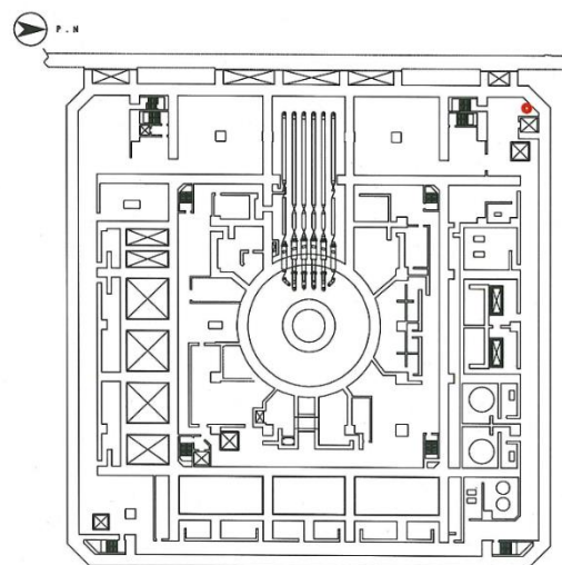
原子燃料処理棟 3F (TP-16100)
