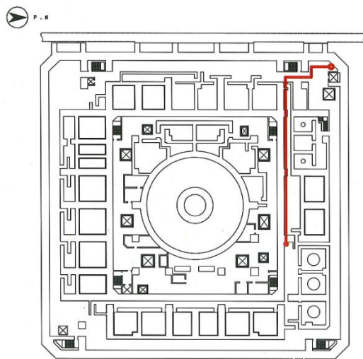
原子燃料処理棟 4F (TP-25100)
