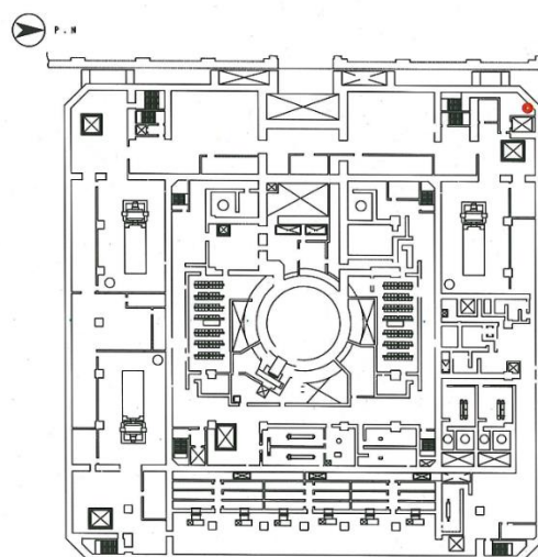
原子燃料処理棟 1F (TP-2700)
