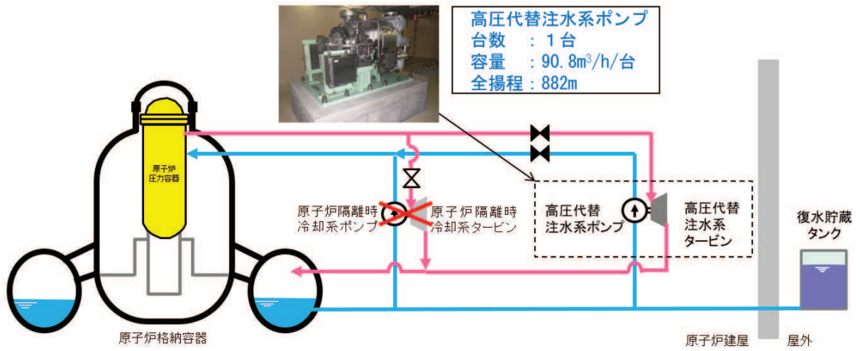
第 57-4-1 図 原子炉隔離時冷却系及び高压代替注水系概略系統図
