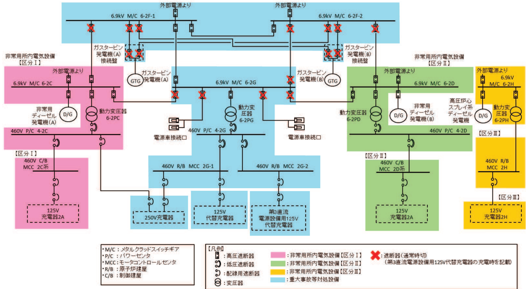
第 57-4-4 図 所内常設直流電源設備（3 系統目）の受電元系統図
