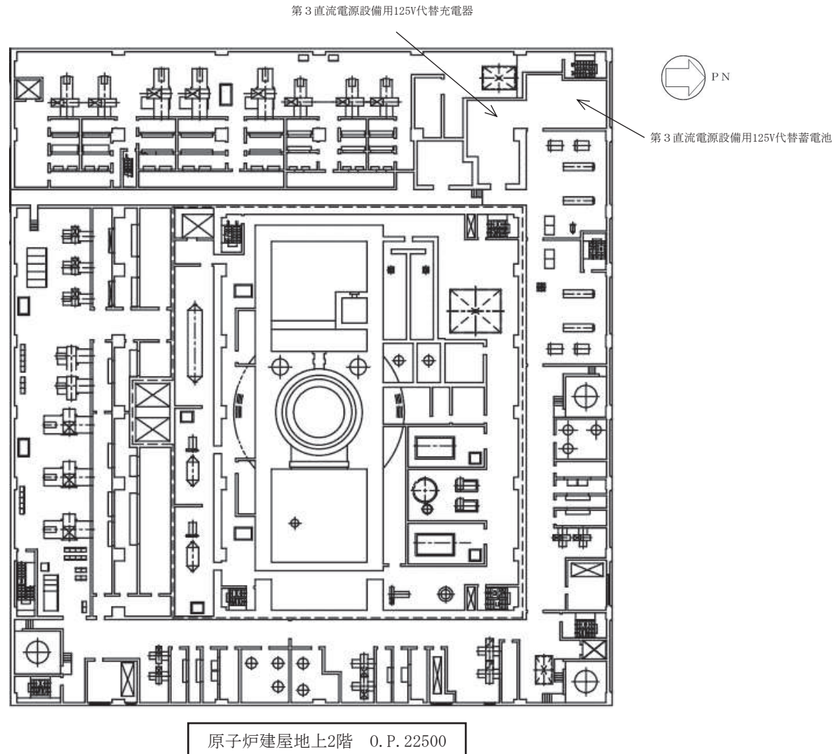
第 57-5-1 図 所内常設直流電源設備（3系統目）設置場所（原子炉建屋地上2階）
