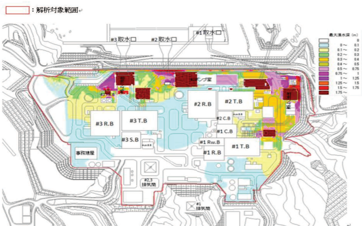
第 57-7-1-1 図 O.P.+33.9m津波による敷地内最大浸水深分布
