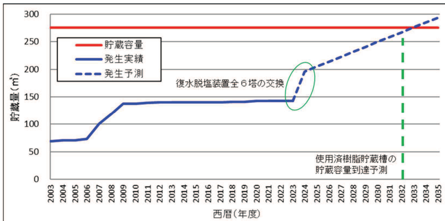
図2-4 使用済樹脂貯蔵槽の貯蔵量予測
