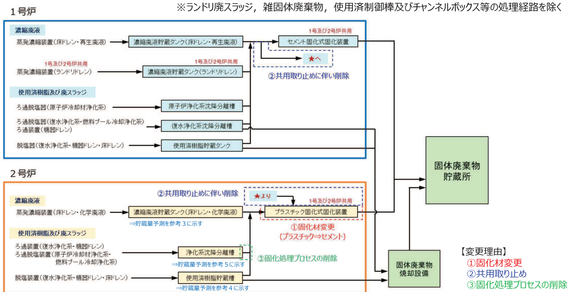
図2-2 女川1号及び2号炉における固体廃棄物処理フロー
