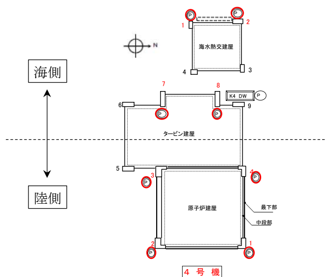
図 12-1 KK4 周辺のサブドレン配置図
