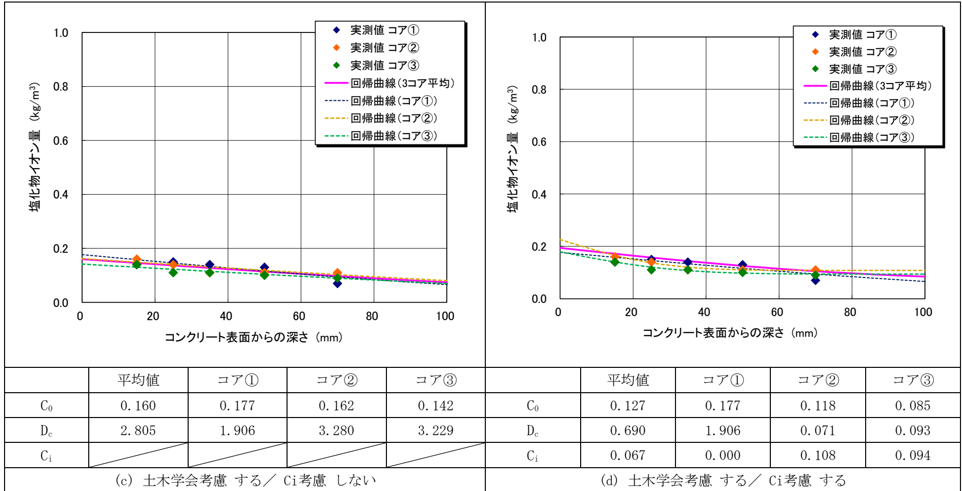
図9-1 (2/2) タービン建屋における回帰分析結果
