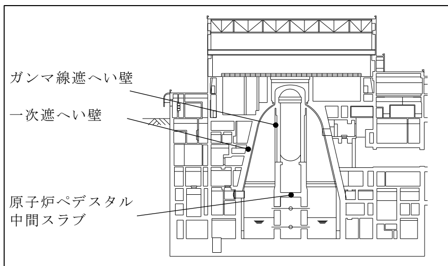
図3 原子炉建屋の概要
