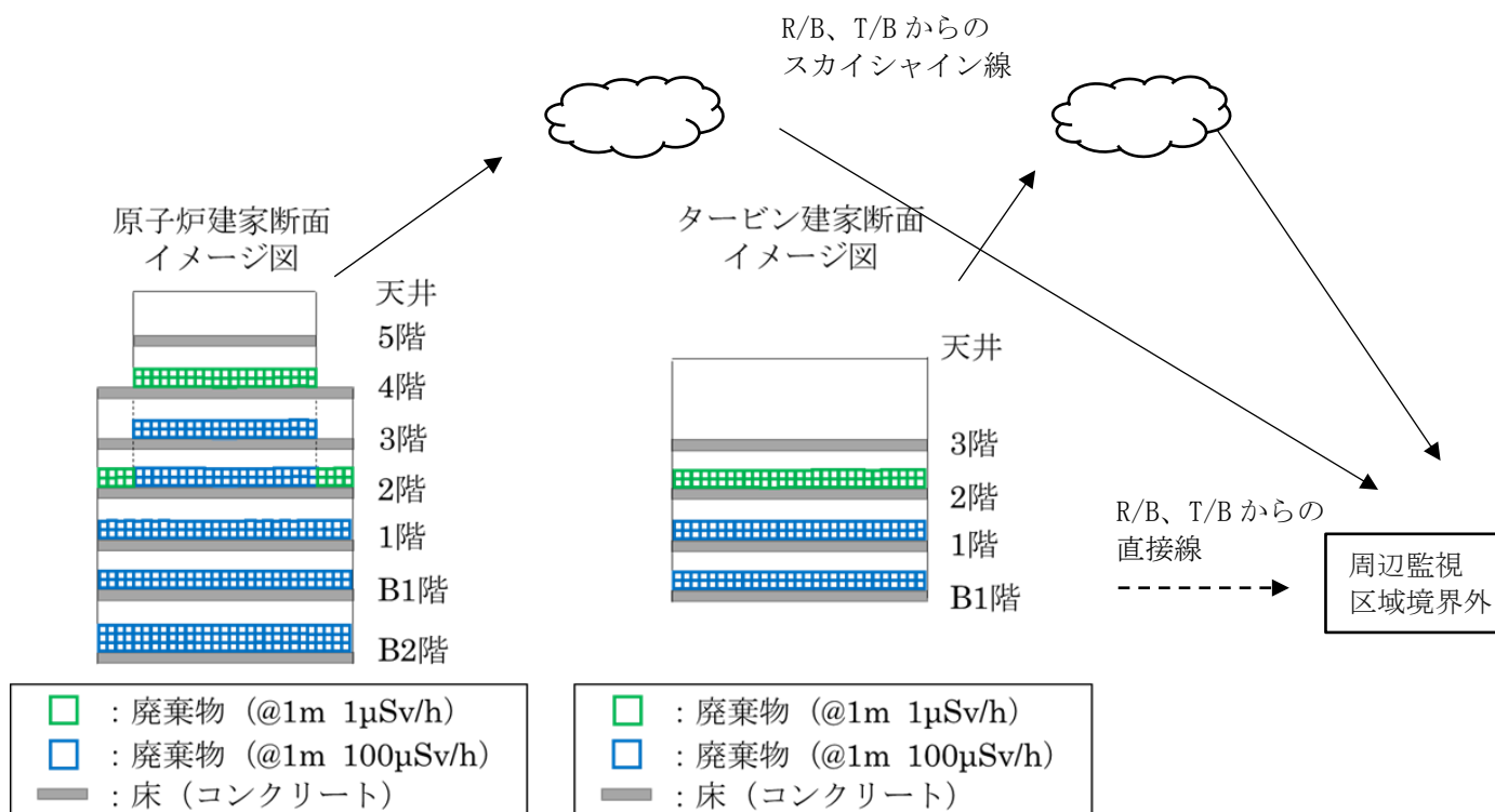
図2 原子炉建屋、タービン建屋評価模式図
