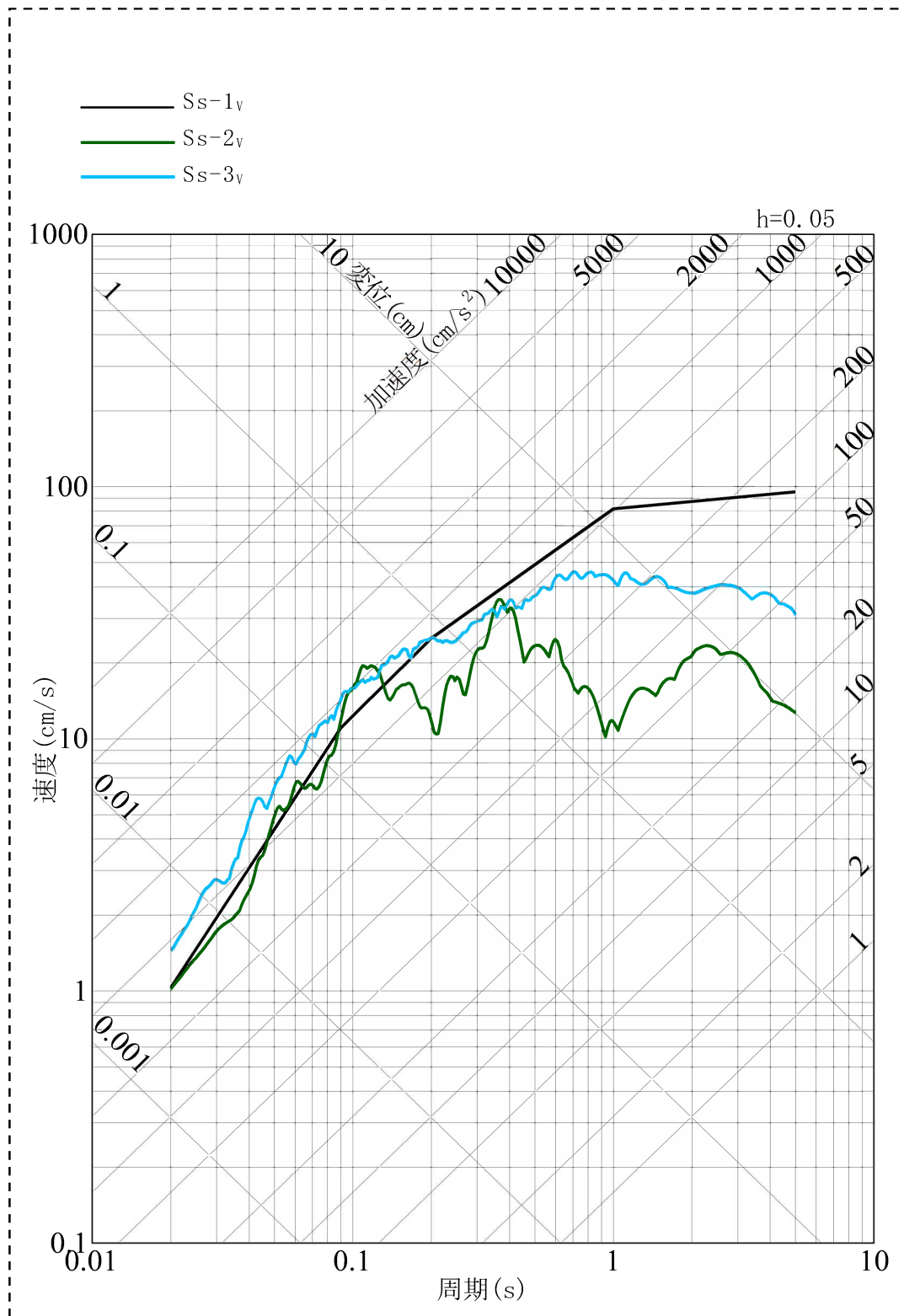
第 5.2 図 基準地震動の応答スペクトル (鉛直方向) 注 1
