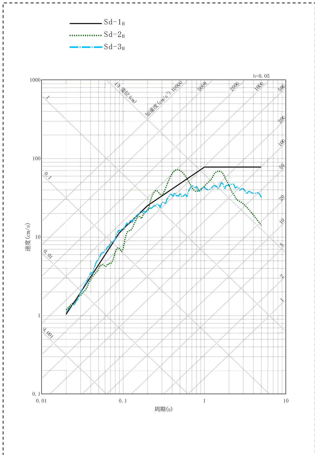
第 1.4.1 図 弾性設計用地震動の応答スペクトル（水平方向） 注 3
