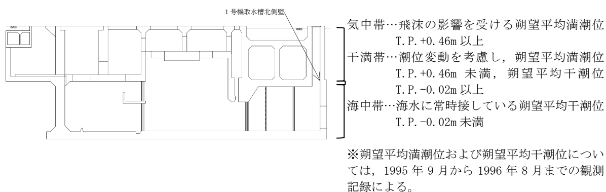
図4 1号機取水槽の概要
