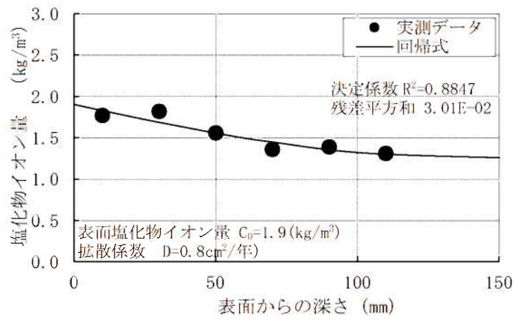
図1(3/9) 取水構造物気中帯 (SP-ci-2u-8) の回帰分析結果 (上：中性化考慮あり [○データを棄却]、下：中性化考慮なし)
