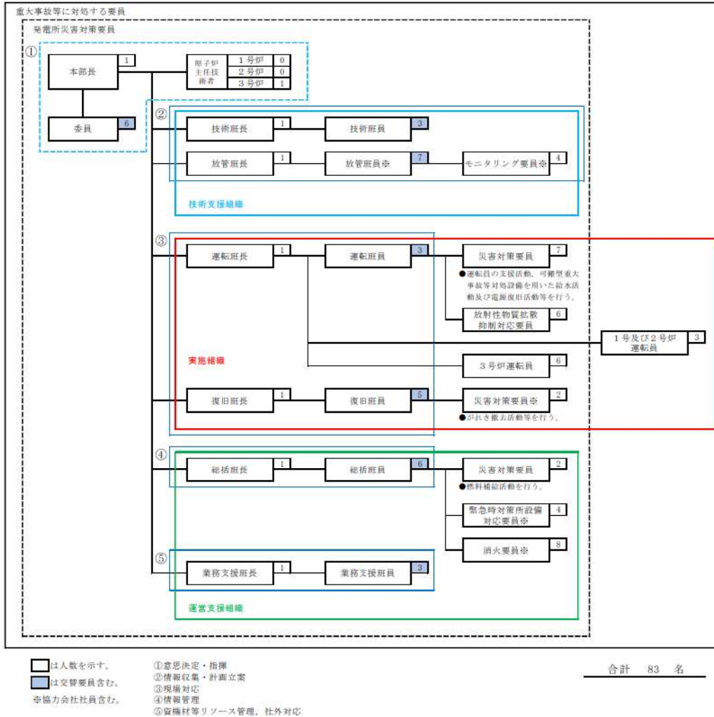
第5図 発電所対策本部体制（プルーム通過時）
