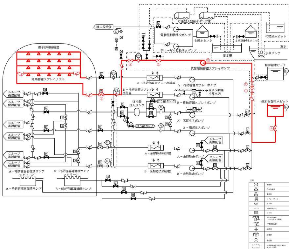
図 49-4-2 代替格納容器スプレィ
