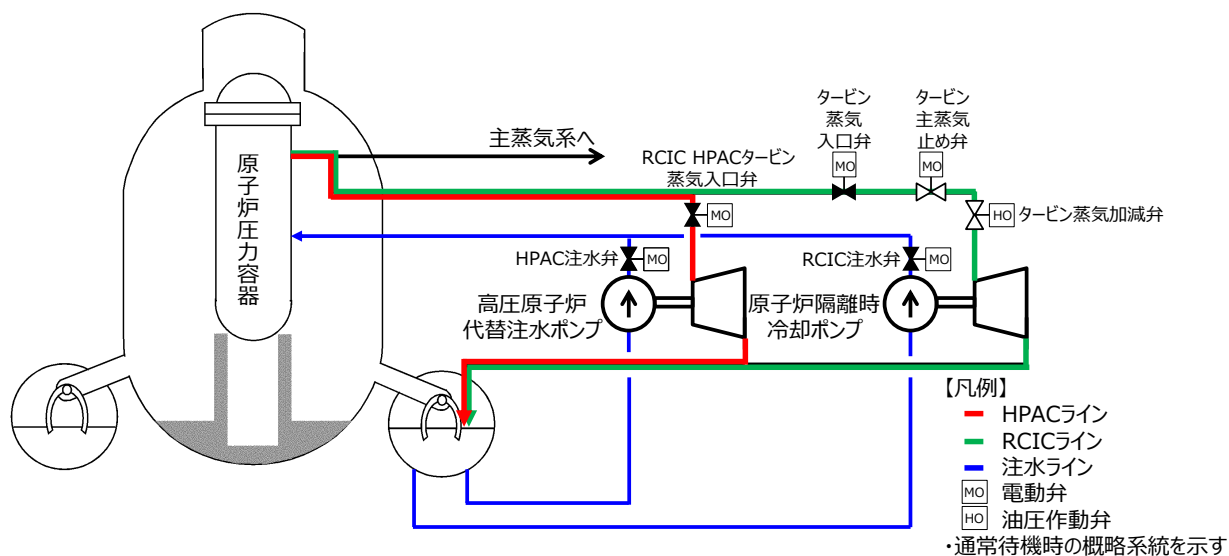
第 57-7-9 図 RCIC 及び HPAC 概略系統図
