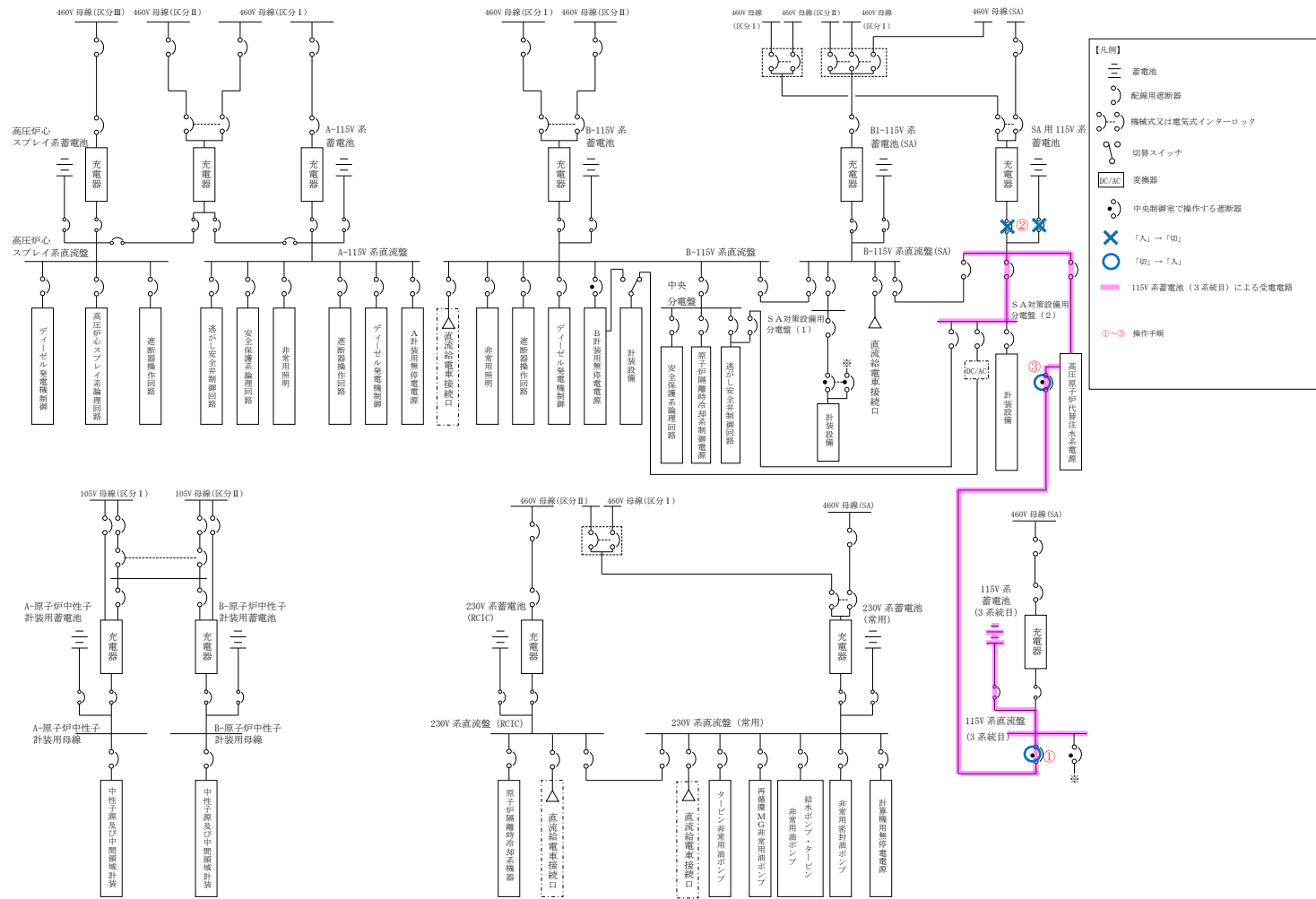
第57-4-2図 所内常設直流電源設備（3系統目）による給電 概要図
