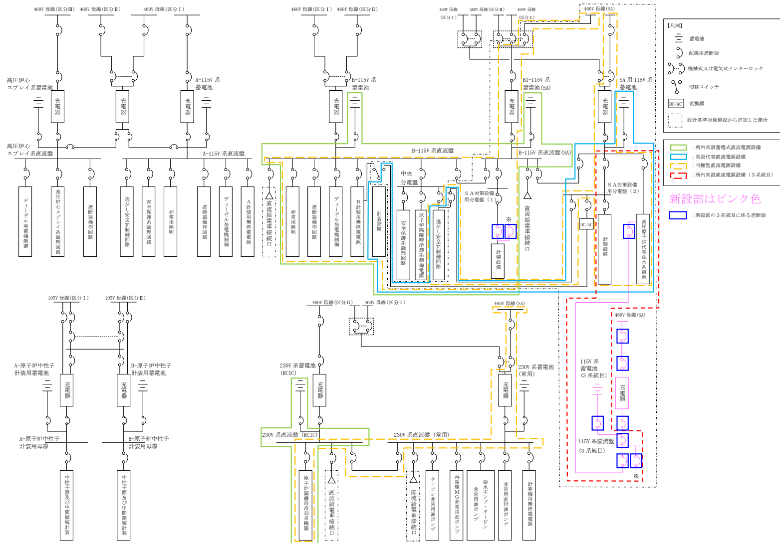
第 41-2-2 図 115V 系蓄電池 (3 系統目) から給電される系統
