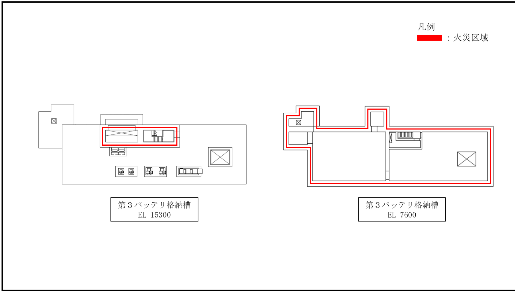
第 41-2-3 図 115V 系蓄電池（3 系統目）を設置する火災区域及び火災区画
