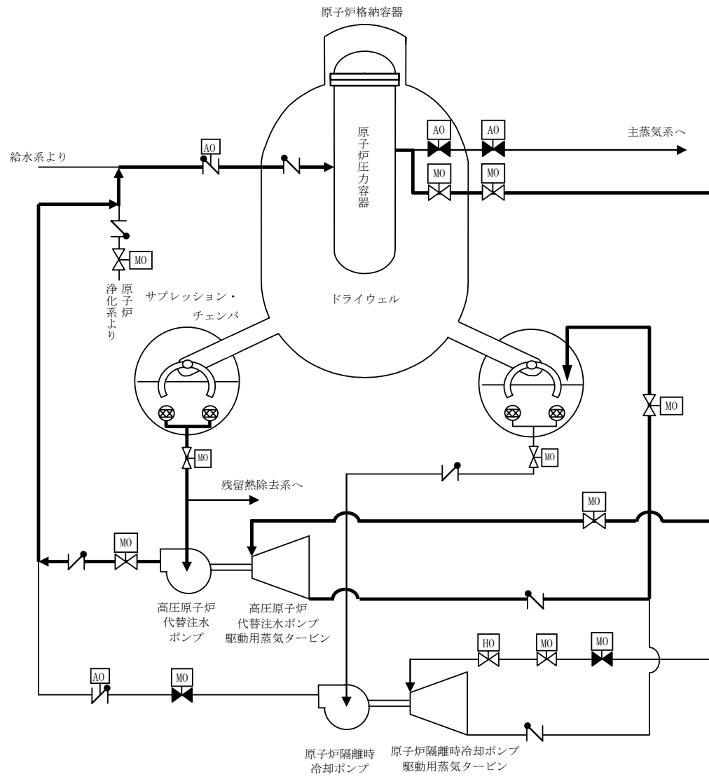
第 57-7-10 図 高圧原子炉代替注水系 系統概要図
