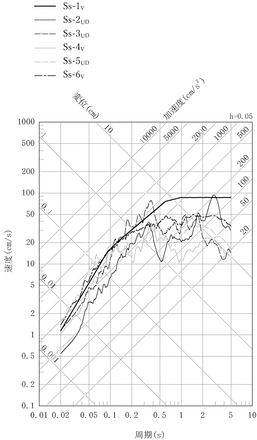
第3-1図 (3/3) Ss-6と現行の基準地震動 Ss-1~5の比較 (鉛直方向)
