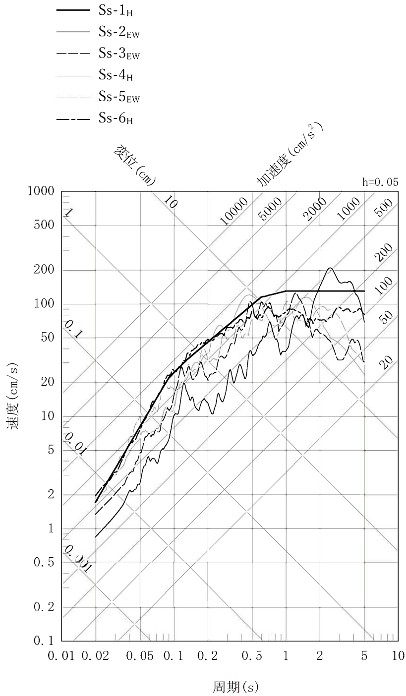
第 3-1 図 (2/3) Ss-6 と現行の基準地震動 Ss-1~5 の比較 (水平[EW]方向)
