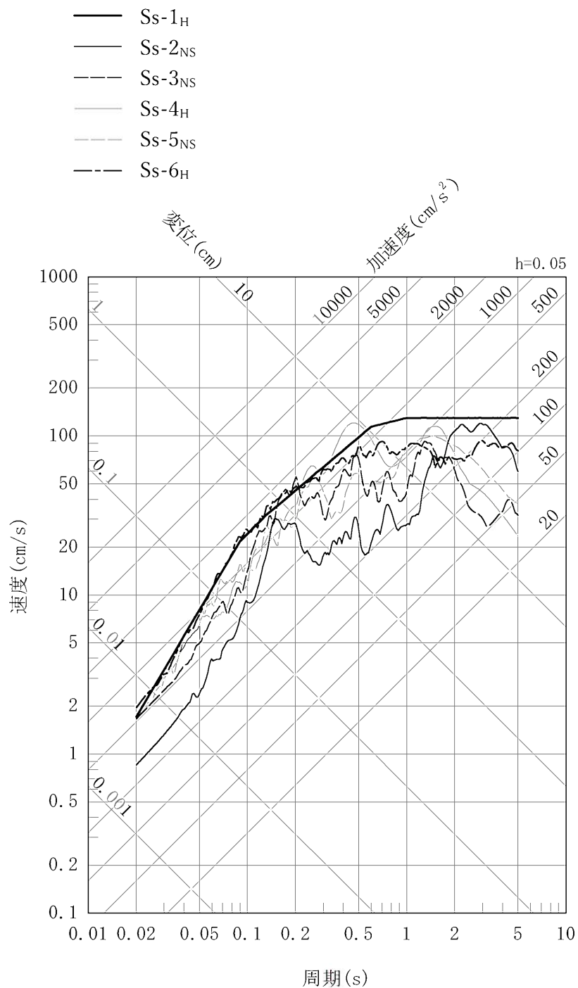
第3-1図 (1/3) Ss-6と現行の基準地震動 Ss-1~5の比較 (水平[NS]方向)
