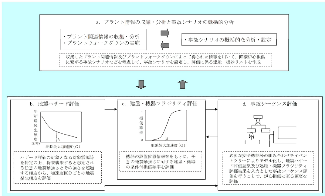
第 3-1 図 地震レベル 1 PRA の評価フロー
