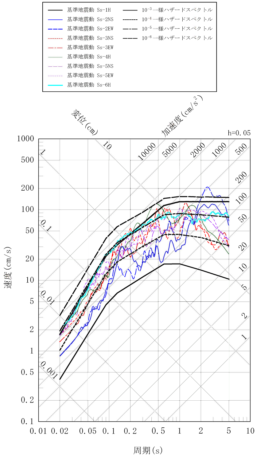
第 3-2 図(1) 基準地震動と一様ハザードスペクトルの比較 (水平方向)
