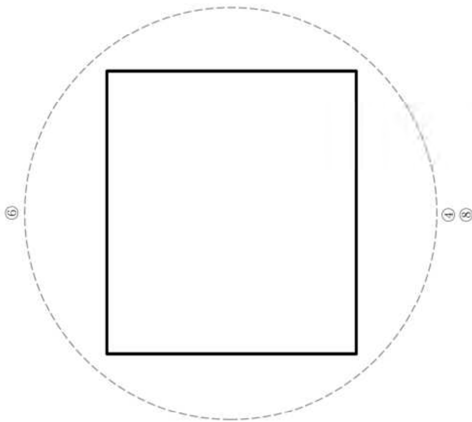
(注) ④、⑤、⑥、⑧の評価点位置は各方向での最大線量当量率となる位置を示している。 別紙5-1図(2/2) 特定兼用キヤスクの表面から1 m離れた位置における代表評価点(水平断面)
