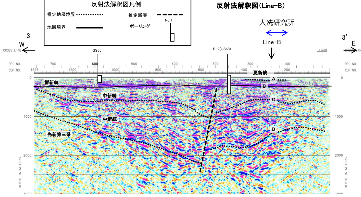
反射法解釈図 (Line-3) 0 2 4 km
