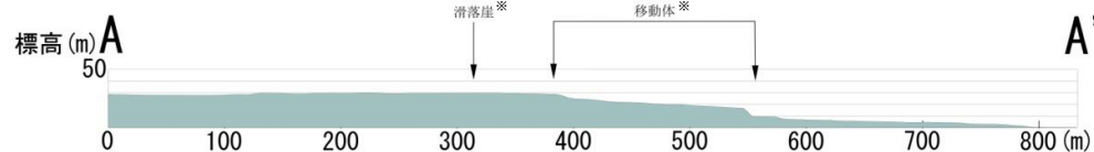
水平:垂直=1:1
