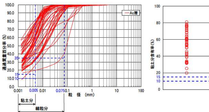
添付 2-3 図 Ac 層の粒度分布，粘土分含有率
