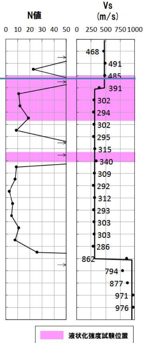
添付 4-8 図 N 値とせん断波速度の比較(RE-5 地点(1, 2 号埋戻土))
