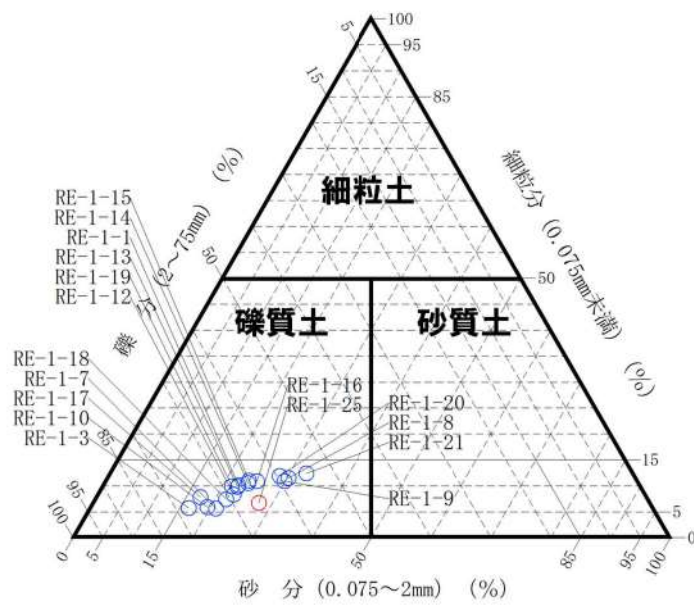
添付 8-13 図 三角座標による分類 (RE-1)
