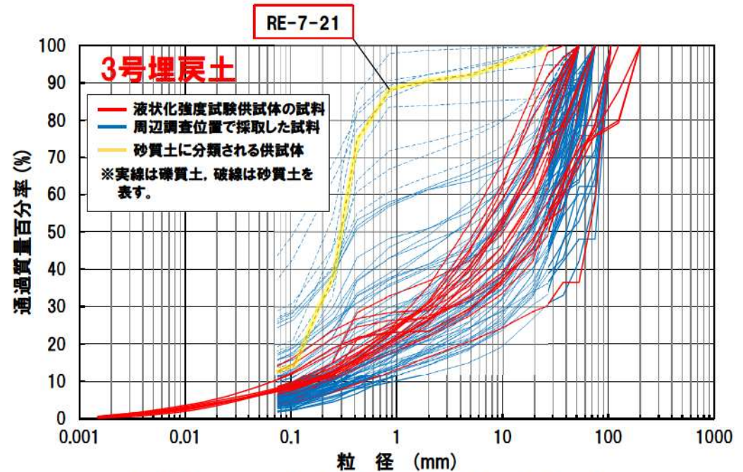
粒径加積曲線
