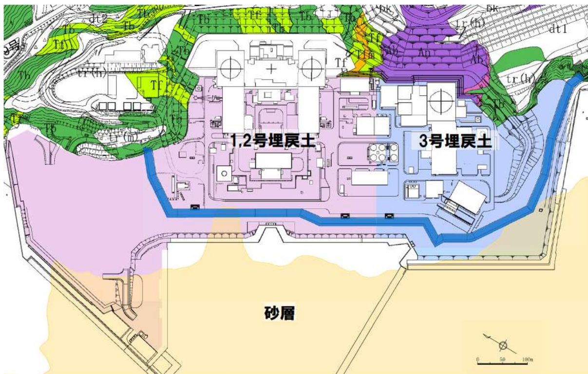
地質平面図
