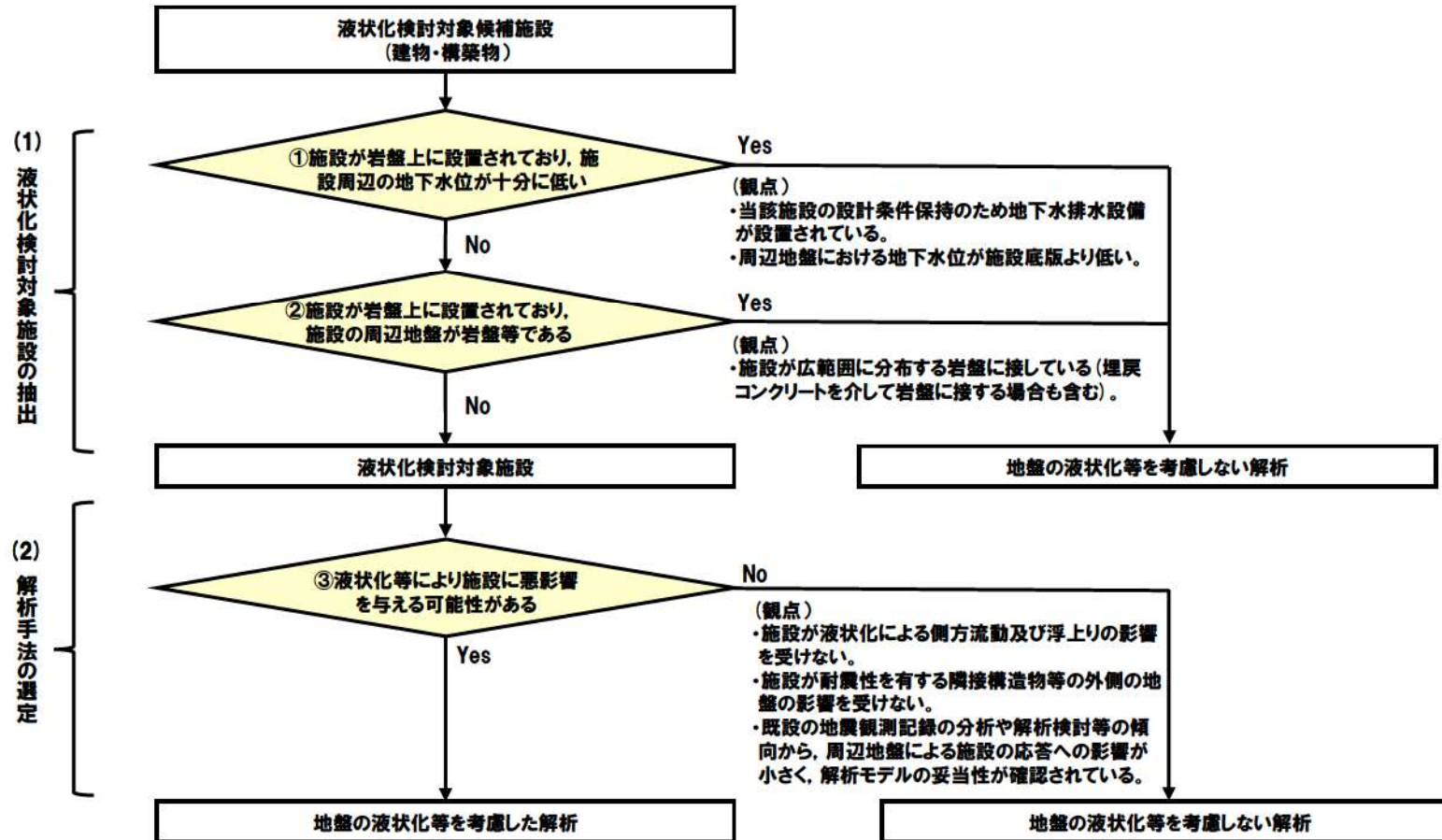
液状化検討対象施設の抽出及び解析手法選定フロー(建物・構築物)
