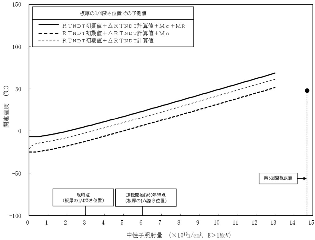
図 4(3/4) 国内脆化予測法による予測と第5回監視試験結果の関係 (母材)
