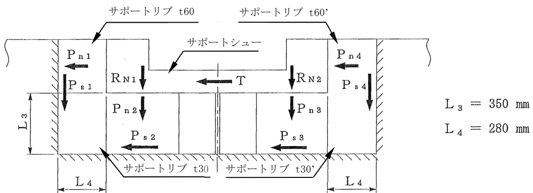
図9-1-4 サポートリブに作用する荷重
