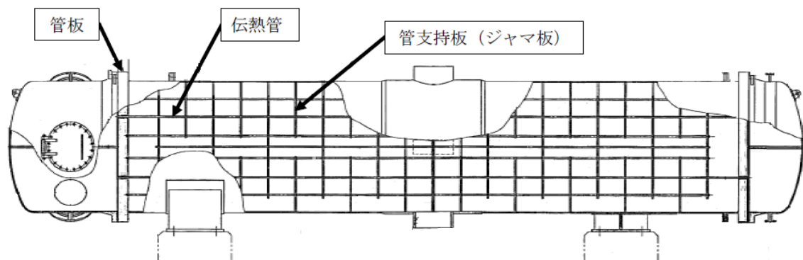
図9-1 原子炉補機冷却水系熱交換器の概略図
