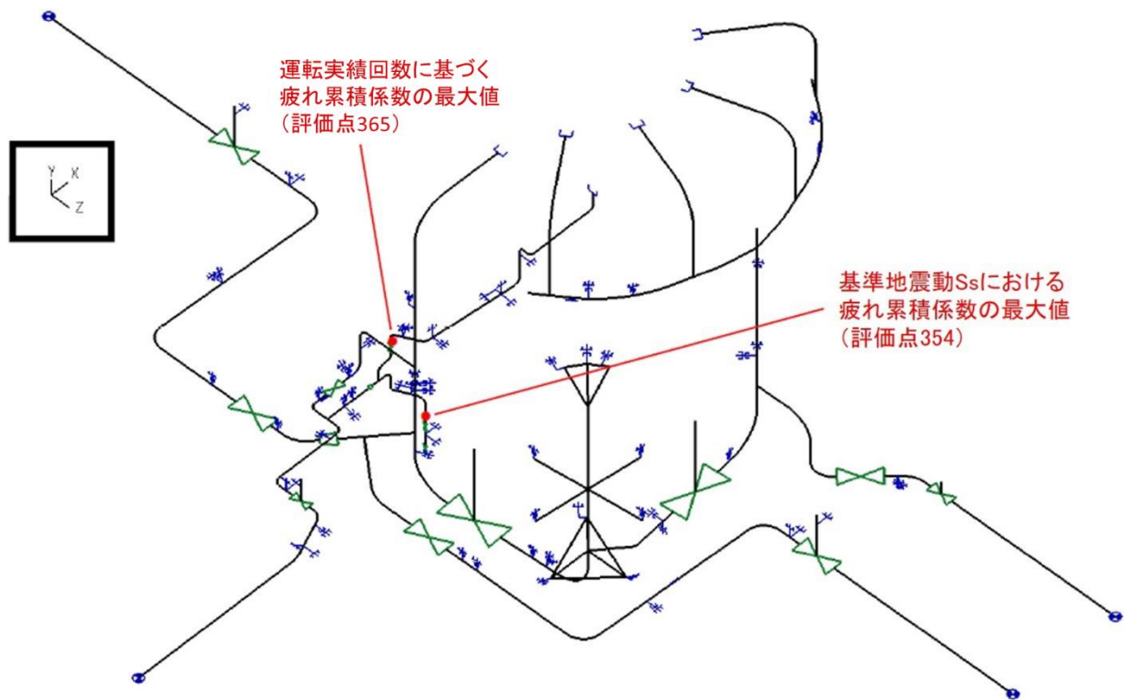
図 6-1 原子炉冷却材浄化系（純水部）配管の疲労解析モデル
