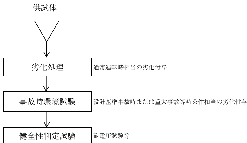
図3.9.5.2-1 長期健全性試験手順および判定方法
