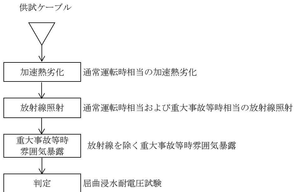
図3.9.5.3-3 難燃PHケーブルの長期健全性試験手順および判定方法
