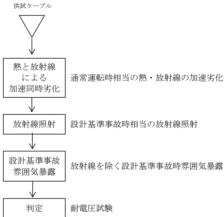
図3.9.5.3-2 難燃PHケーブルのACAガイドに基づく試験手順
