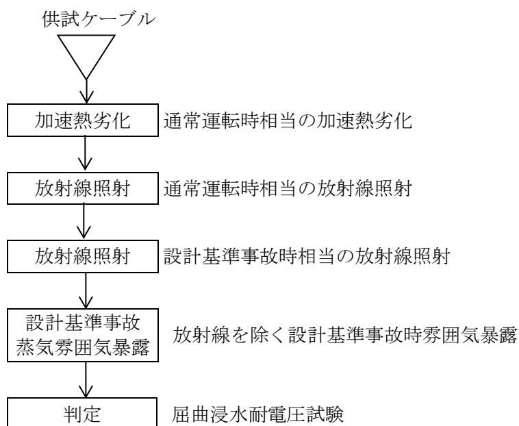
図3.9.5.3-1 難燃PHケーブルの長期健全性試験手順および判定方法
