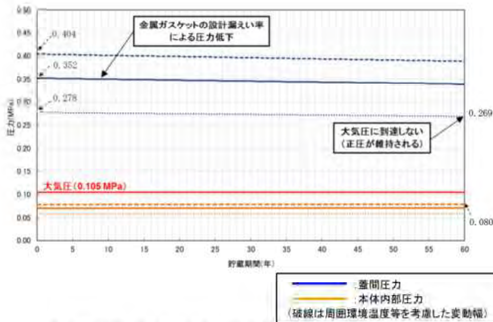
金属ガスケットの設計漏えい率による蓋間圧力の経時変化の例
