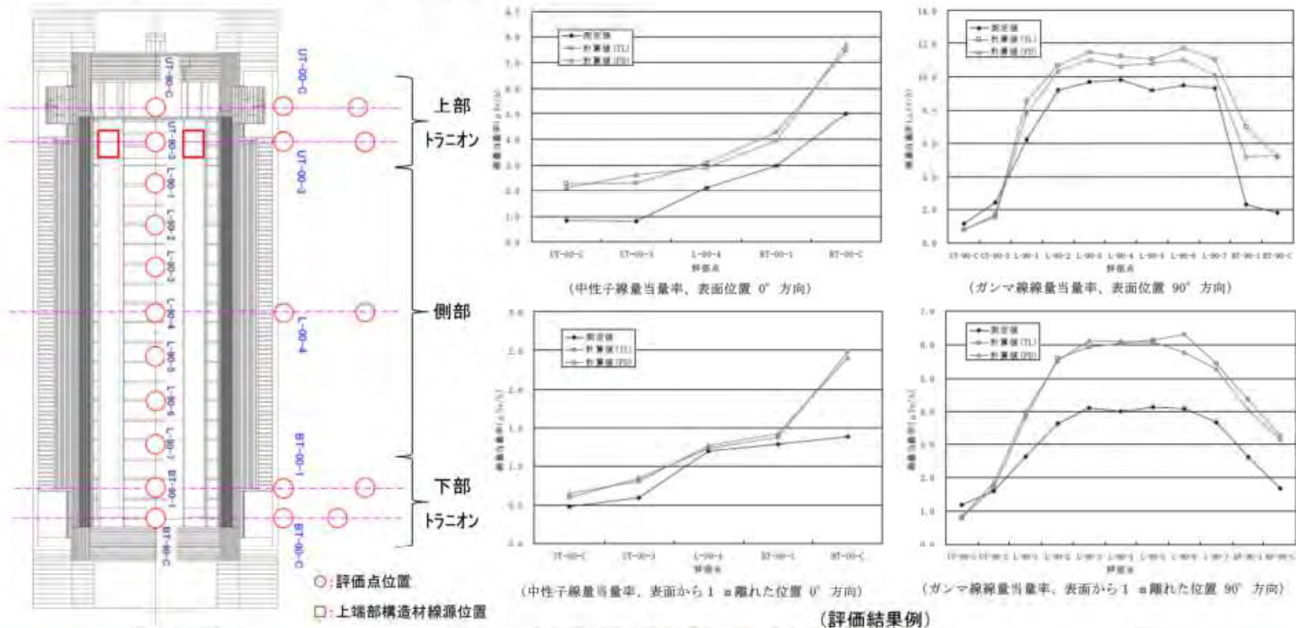
NFT-14P型輸送容器によるMCNP5コードの検証 (出典) 一般社団法人日本原子力学会「モンテカルロ法による放射性物質輸送容器の遮蔽安全評価手法の高度化 平成23年度報告書」(2012)
