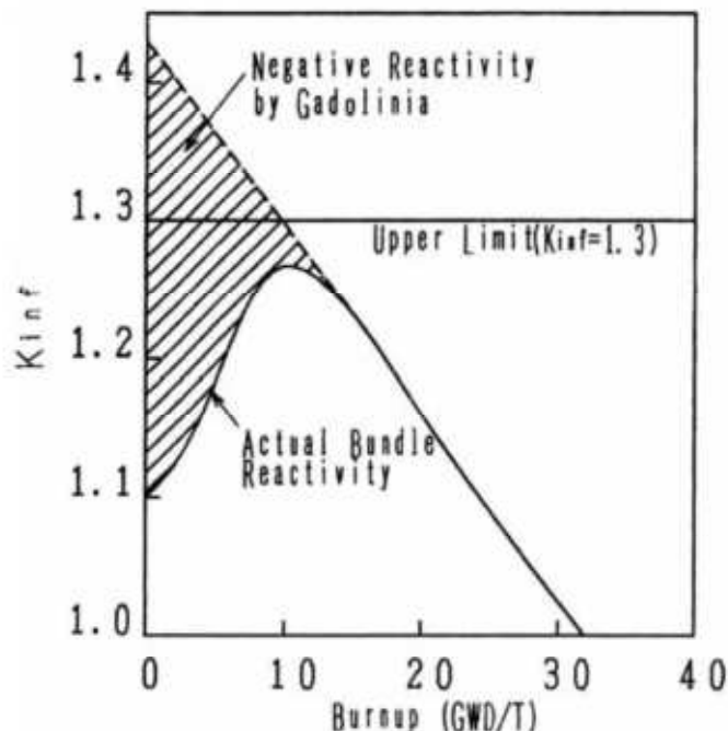
BWR燃料集合体の反応度特性
