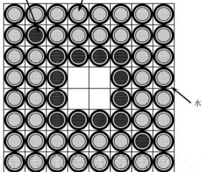
冠水時臨界解析における燃料棒配置
