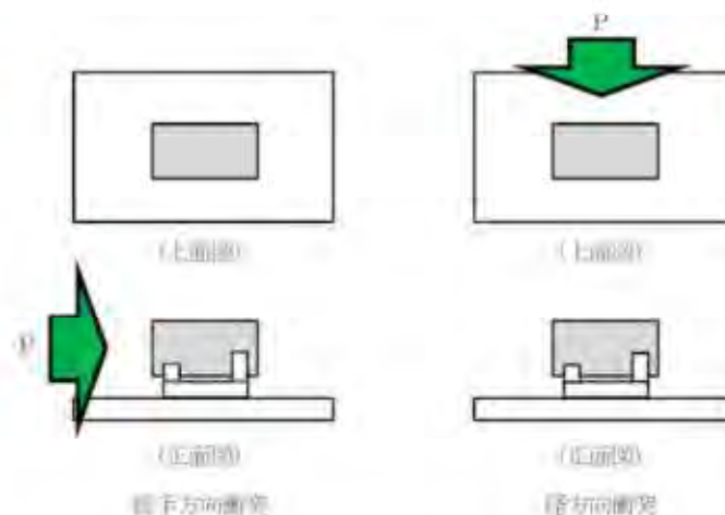
津波荷重の作用方向
