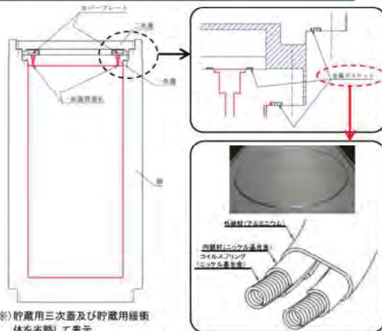
閉じ込め構造図
