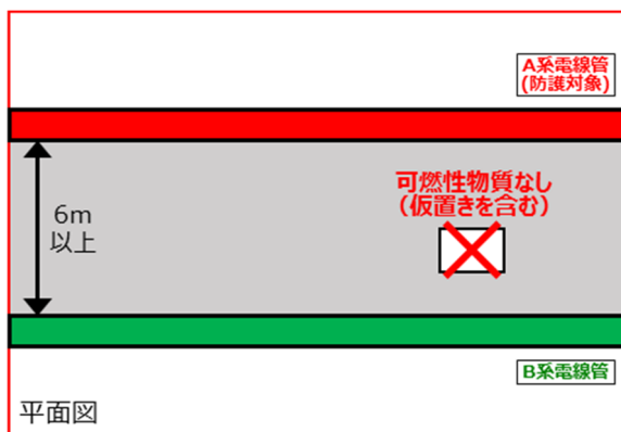
第 1-1-2 図 b. における隔離設計イメージ
