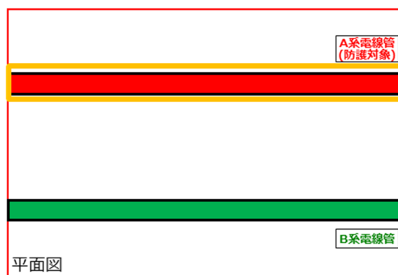
第 1-1-3 図 c. における隔壁設計イメージ
