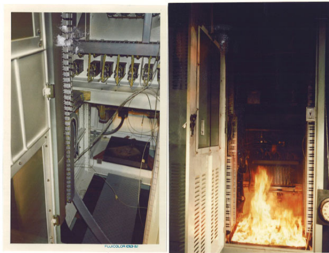
第 1-3-2 図 試験の実施状況
