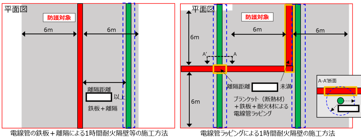
第 1-1-10 図 分離対象が異なる系列の電線管等の場合の隔壁等施工方法 (例)
