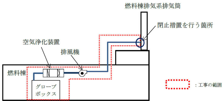
図1 燃料棟排気系統概略図
