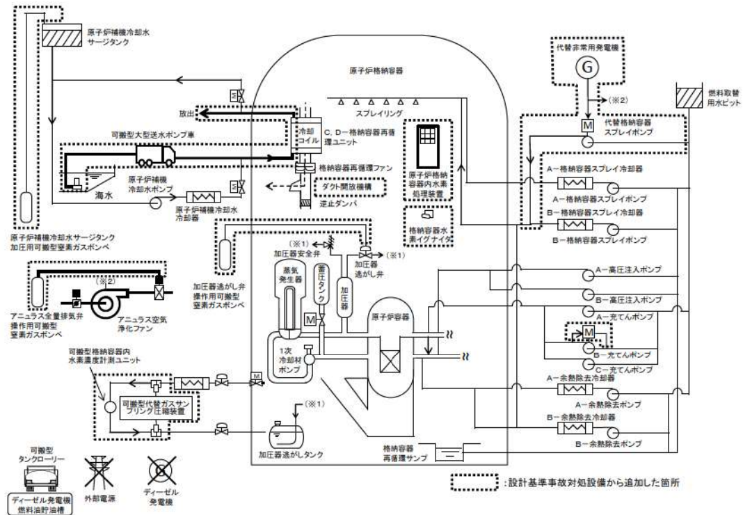
第 7.2.1.2.1 図 「雰囲気圧力・温度による静的負荷（格納容器過温破損）」
