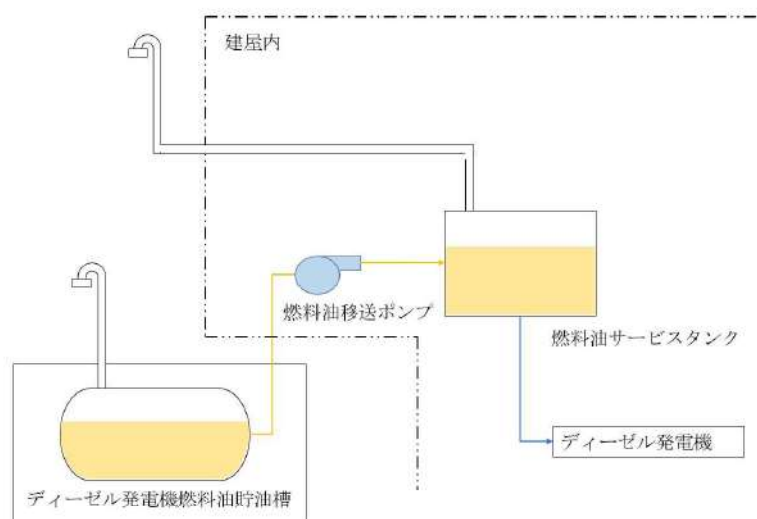
第 1-24 図：油タンクのベント管設置の概要
