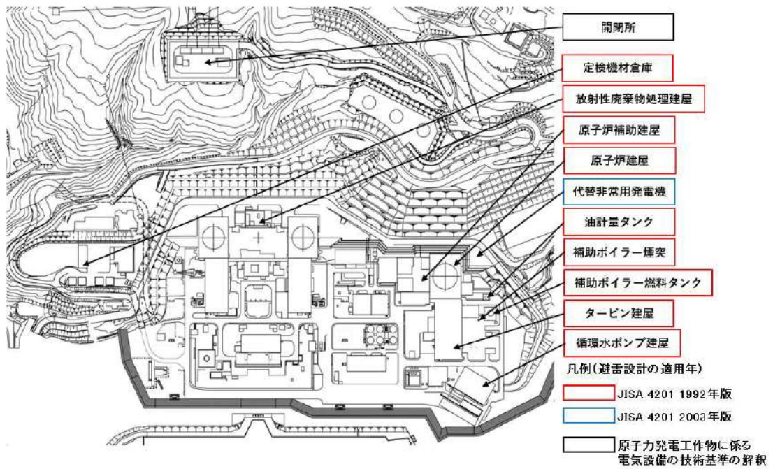
第 1-11 図：避雷設備の設置対象建屋等
